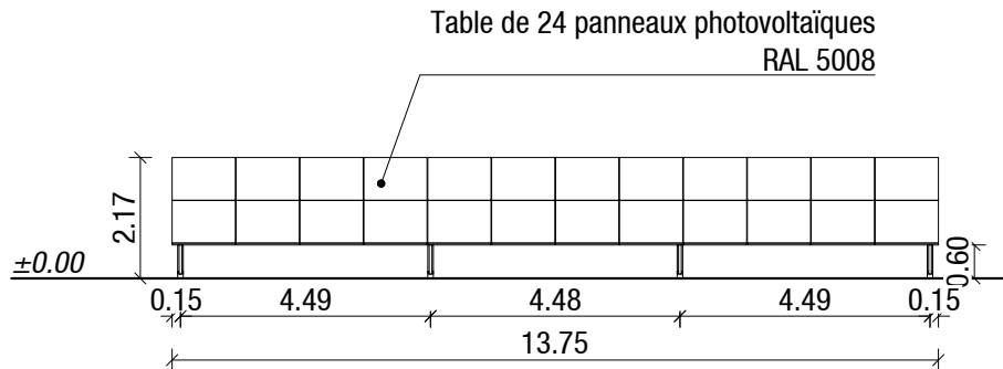
FAÇADE SUD
