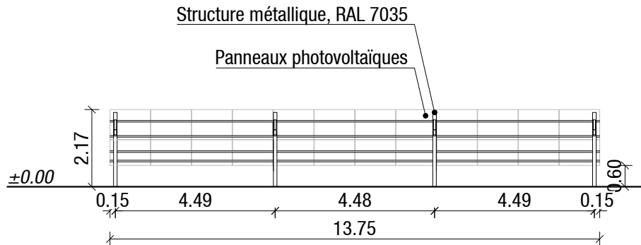
FAÇADE NORD
