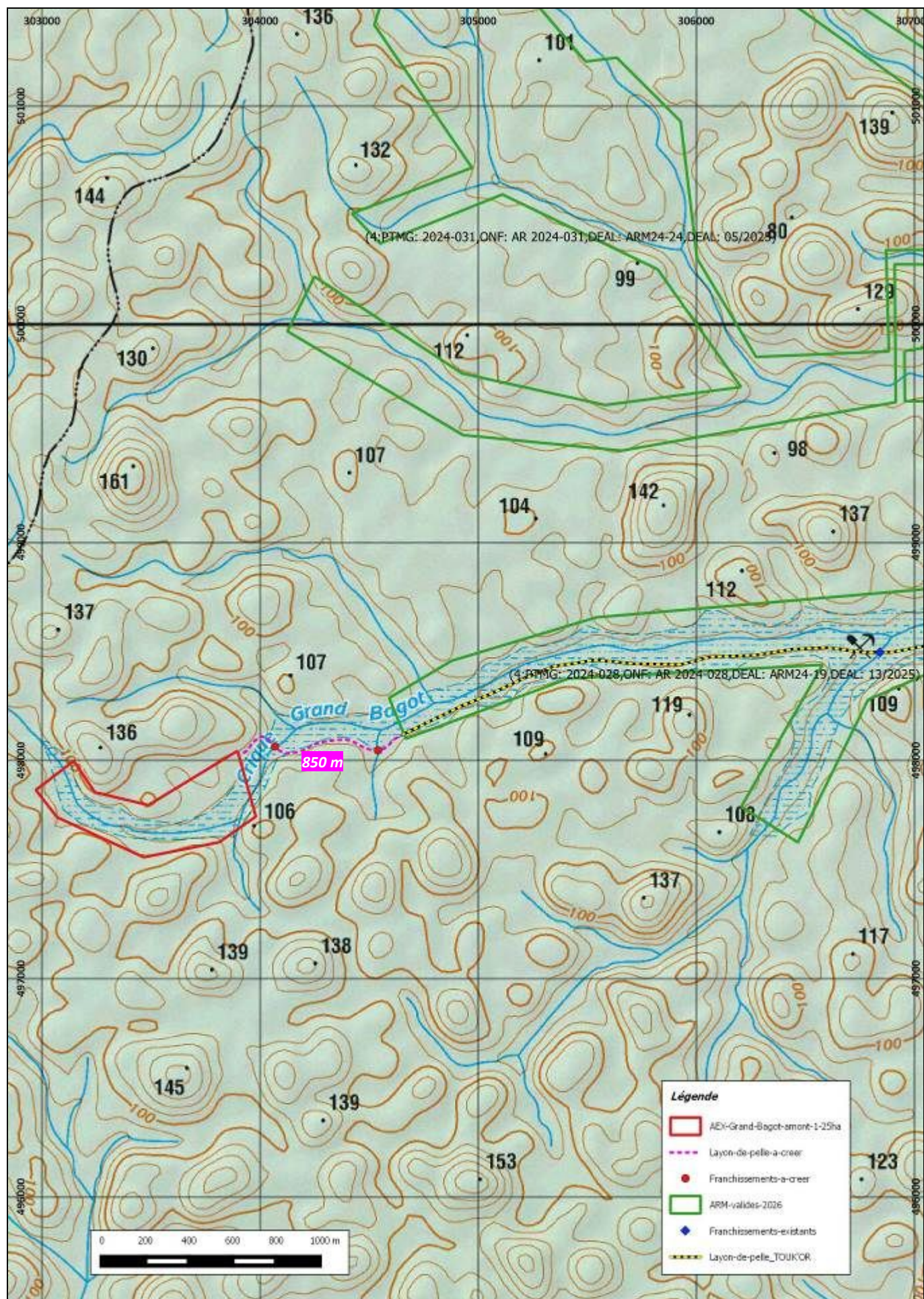
Plan de projet dans le cadre de l'AEX « Amont Grand Bagot 1 » de l'entreprise FERNANDES COSTA sur un fond de carte IGN adapté au 1/20 000° en RGFG95 UTM22
