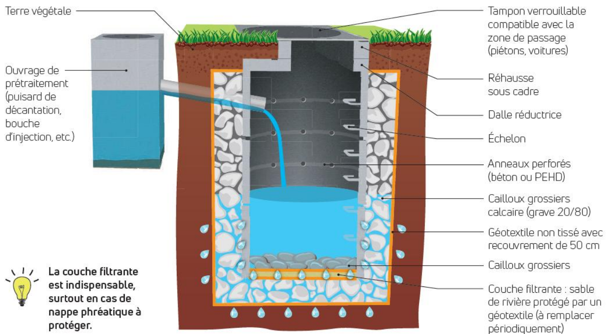
Figure 10: Le puits d'infiltration (ADOPTA)
