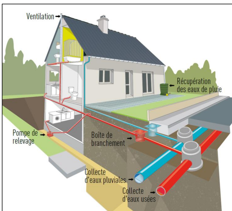
Figure 2 : Schéma de principe de l'assainissement collectif
