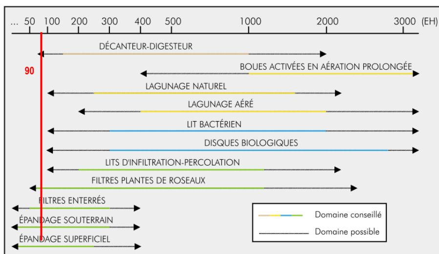
Figure 6 : Domaines d'utilisation des filières type (Source : FNDAE 22)
