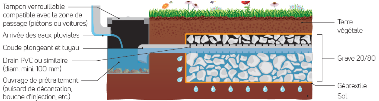
Figure 9: Tranchée d'infiltration (ADOPTA)
