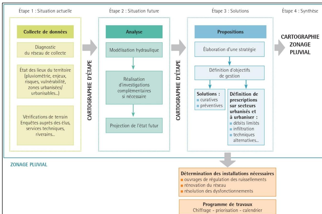
Figure 3 : Démarche d'élaboration d'un zonage pluvial (Cerema, 2020)
