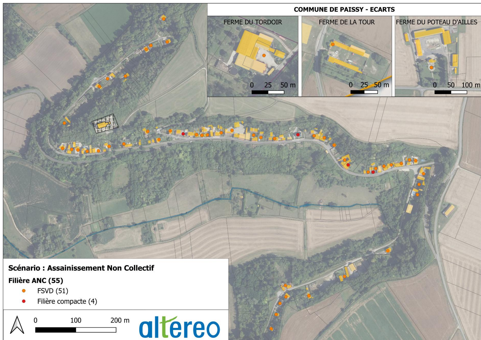
Figure 11 : Cartographie de la solution 2
