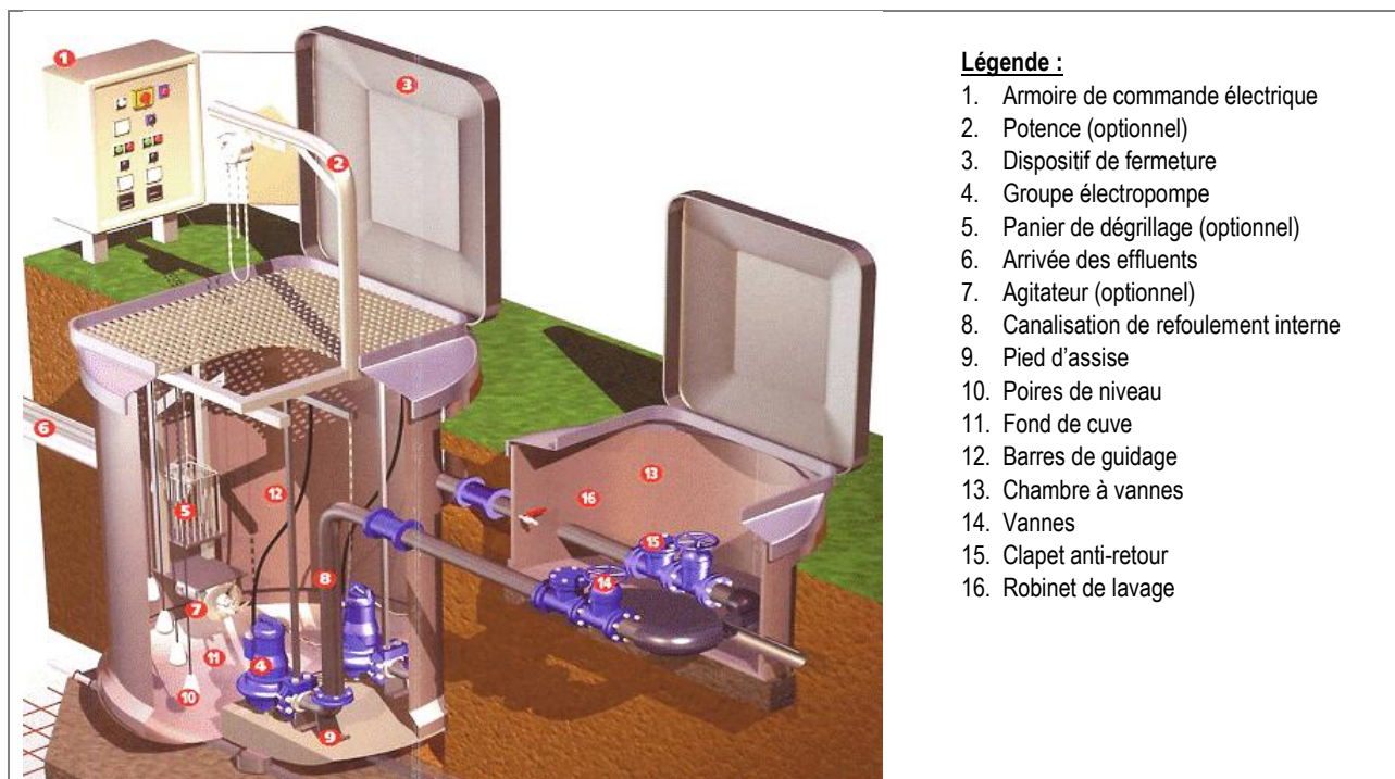
Figure 4 : Schéma de principe d'un poste de refoulement
