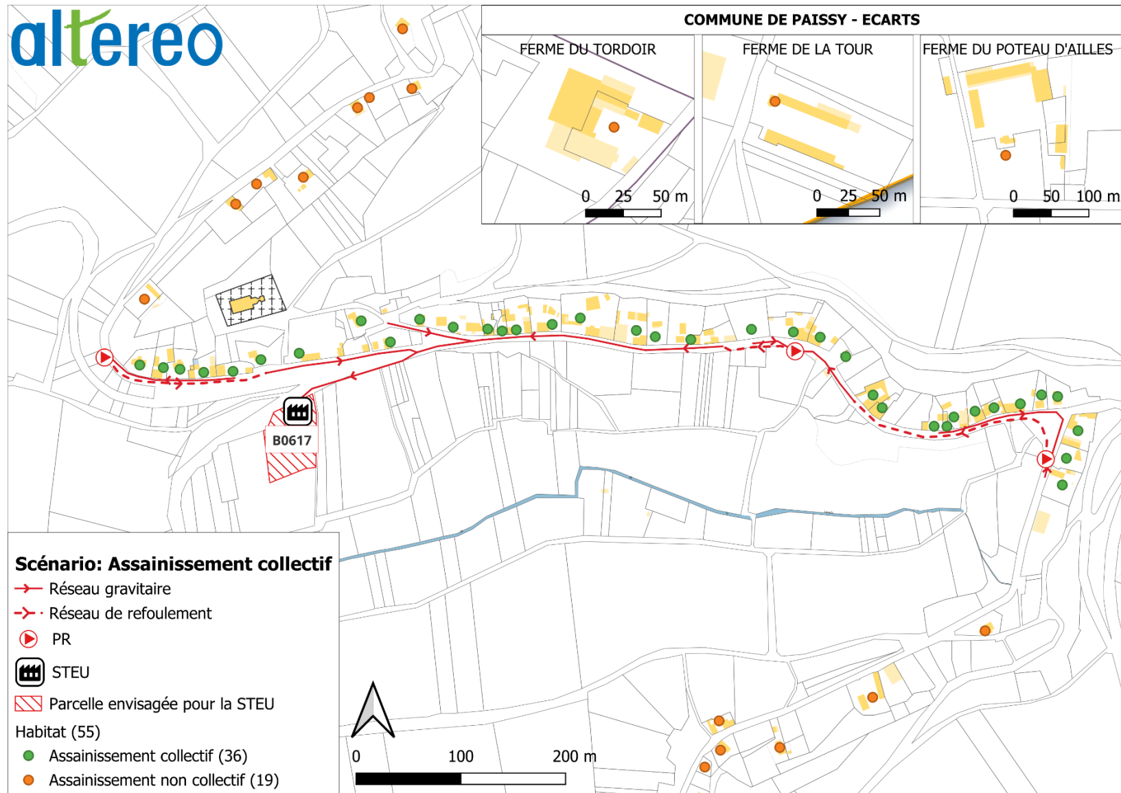
Figure 10 : Cartographie de la solution 1
