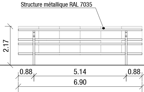
FAÇADE NORD
