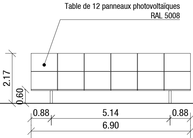
FAÇADE SUD
