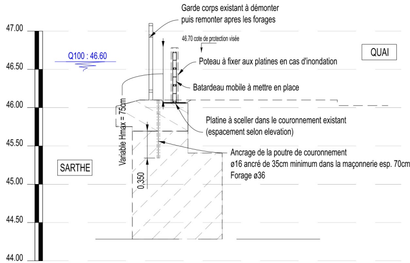
COUPE TYPE SOLUTION C
