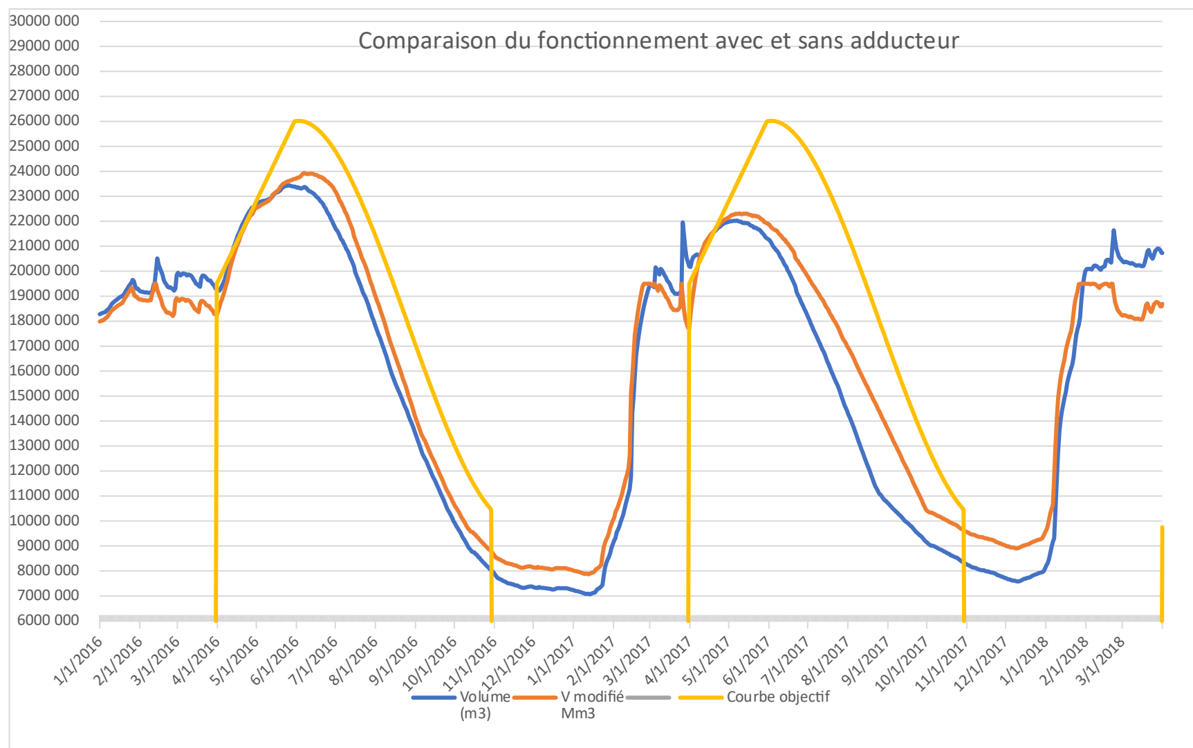
e 9 : Comparaison graphique des données d'exploitations et de l'utilisation de l'adducteur sur la période 2016-2017 – scénario 2
