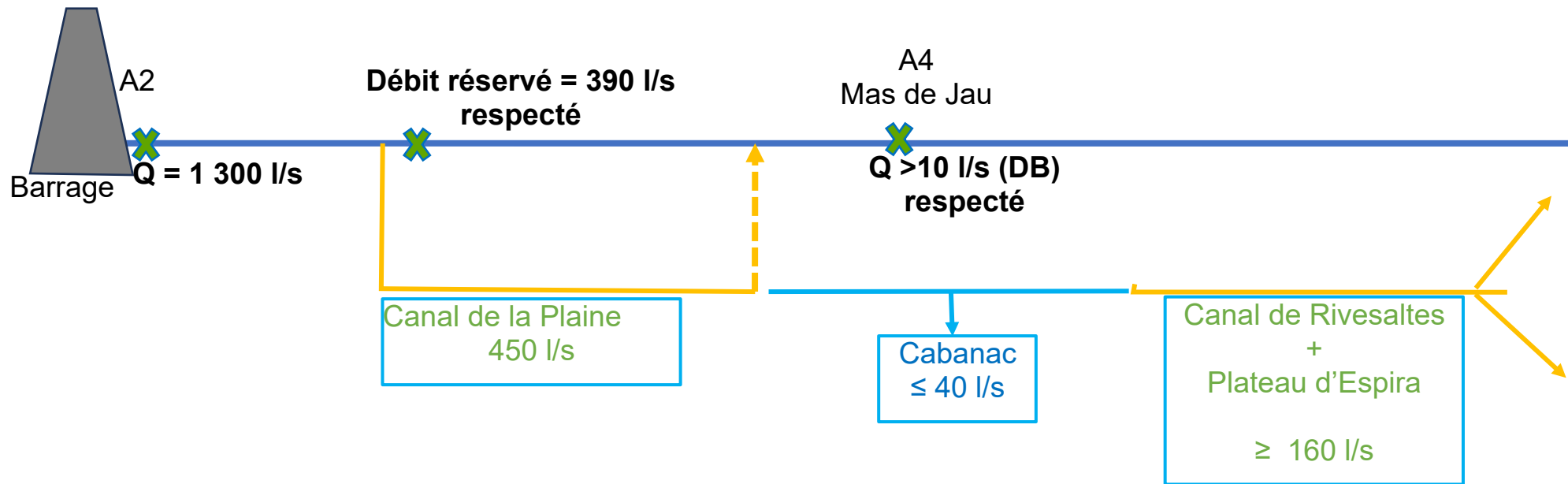
Figure 4 : schéma de l'organisation des débits en aval du barrage en cas de fonctionnement de l'adducteur
