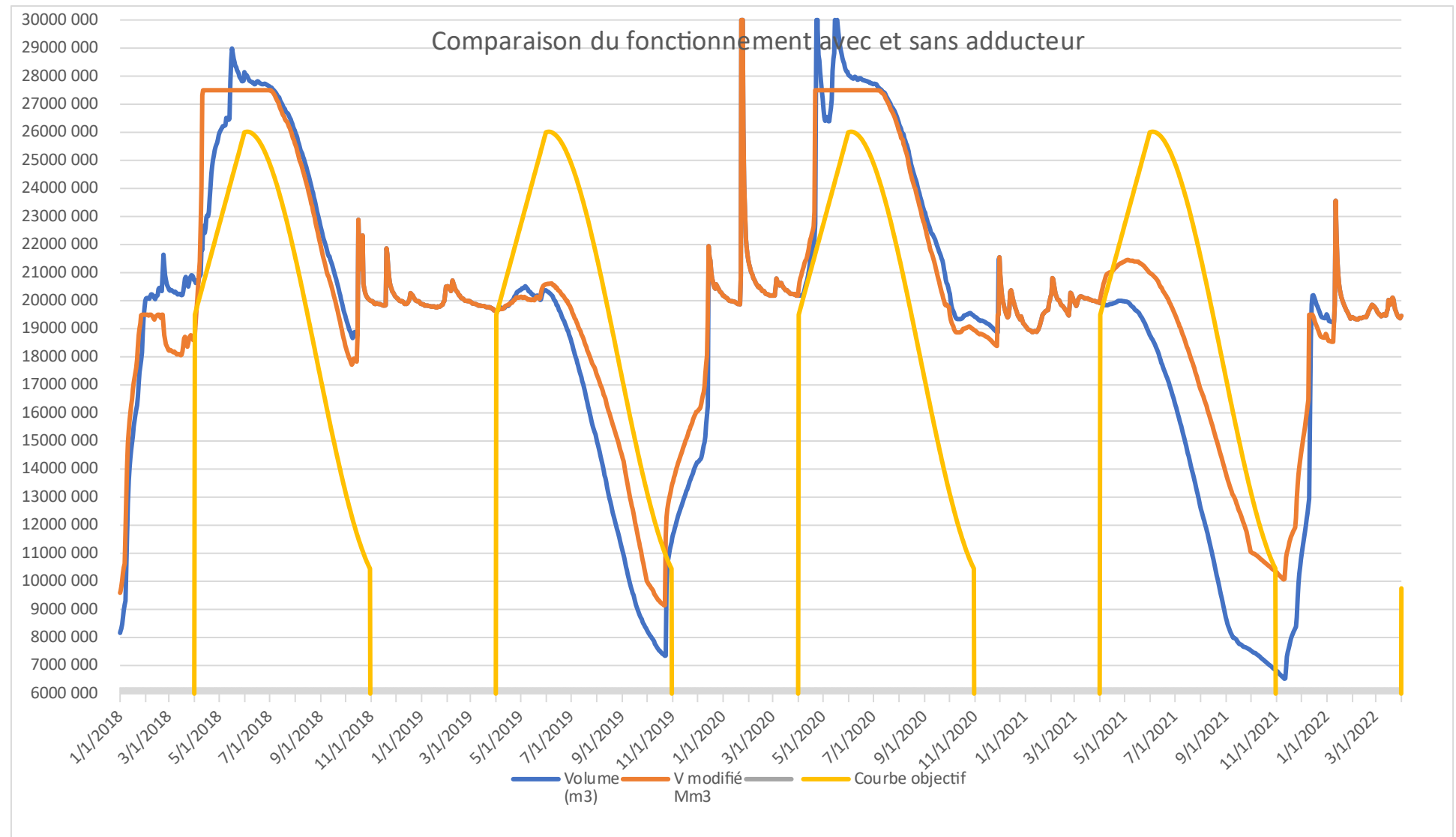
Figure 10 : Comparaison graphique des données d'exploitations et de l'utilisation de l'adducteur sur la période 2018-2021 – scénario 2
