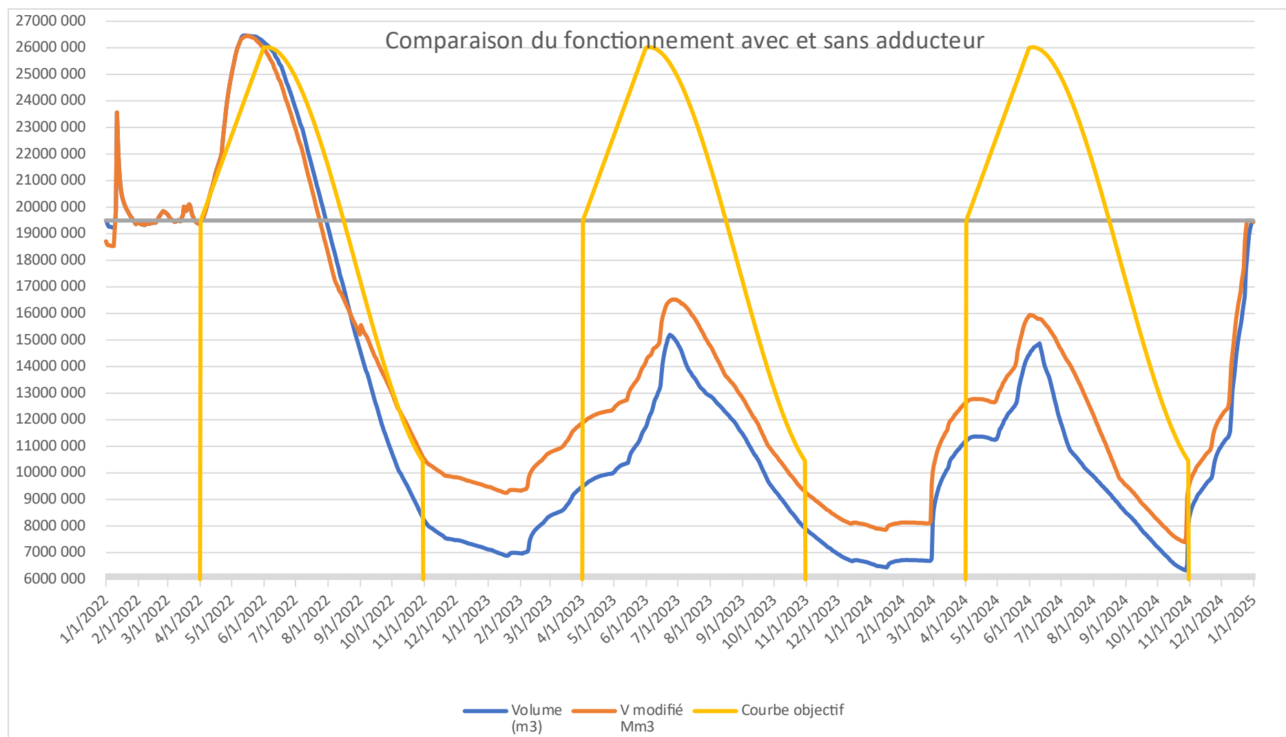
Figure 7 : Comparaison graphique des données d'exploitations et de l'utilisation de l'adducteur sur la période 2022-2024 – scénario 1
