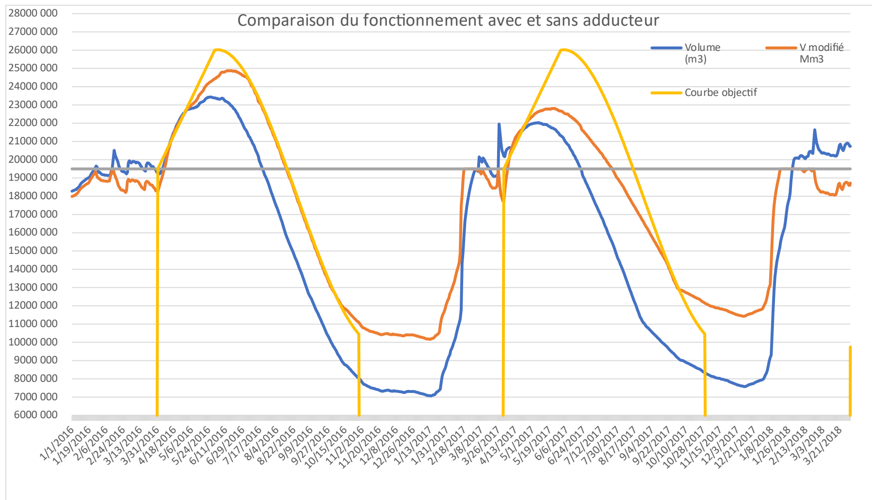
Figure 5 : Comparaison graphique des données d'exploitations et de l'utilisation de l'adducteur sur la période 2016-2017 – scénario 1
