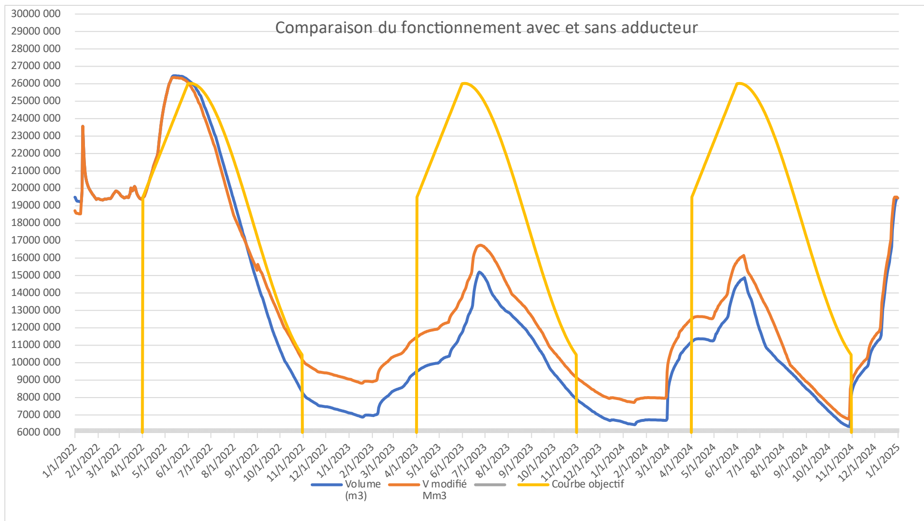
Figure 11 : Comparaison graphique des données d'exploitations et de l'utilisation de l'adducteur sur la période 2022-2024 – scénario 2
