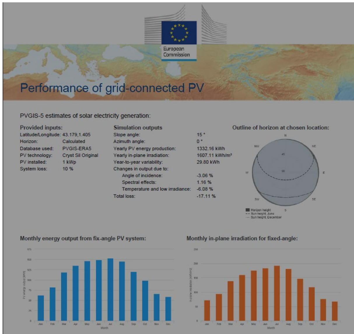
Figure 7 : Etude du gisement – Source : PVGIS
