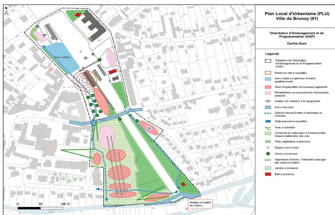
Figure 3: Schéma d'aménagement de l'OAP n° 12 « Centre-Gare » (OAP p.155).
