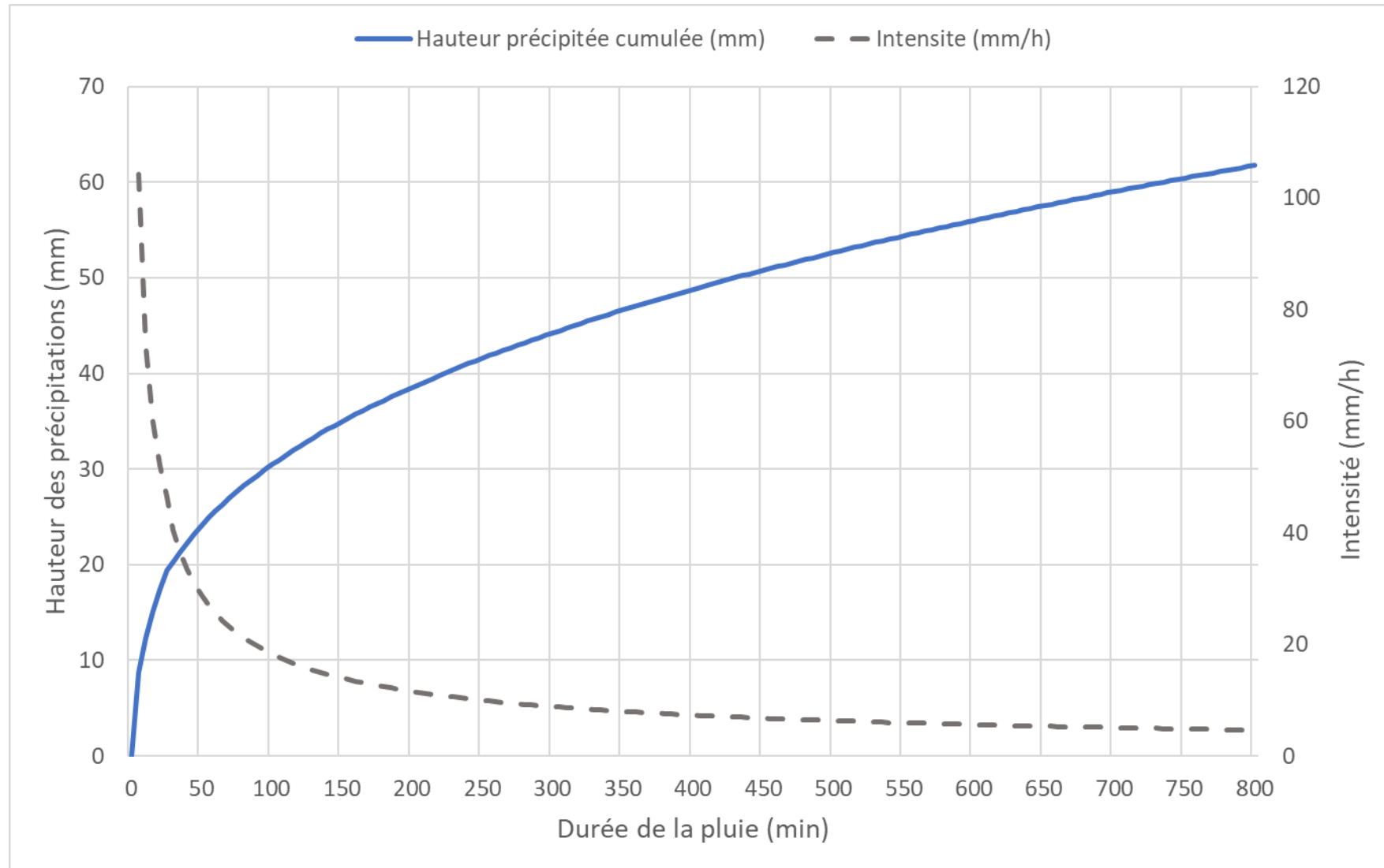
Figure 13 – Caractéristiques de la pluie de projet (occurrence décennale)
