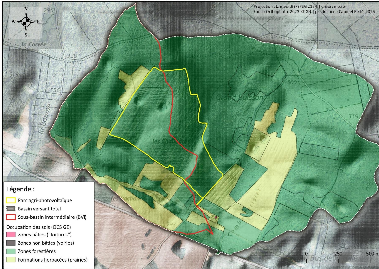
Figure 9 – Cartographie des surfaces actives du bassin versant AVANT aménagement.
