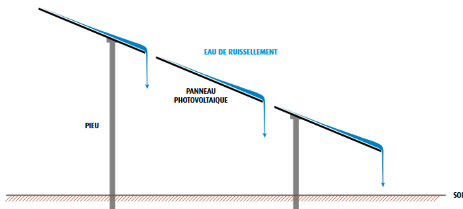
Figure 7 - Schéma montrant l'effet des modules photovoltaïques sur l'écoulement des eaux de pluies (source : MEDDTL, Guide de l'étude d'impact).
