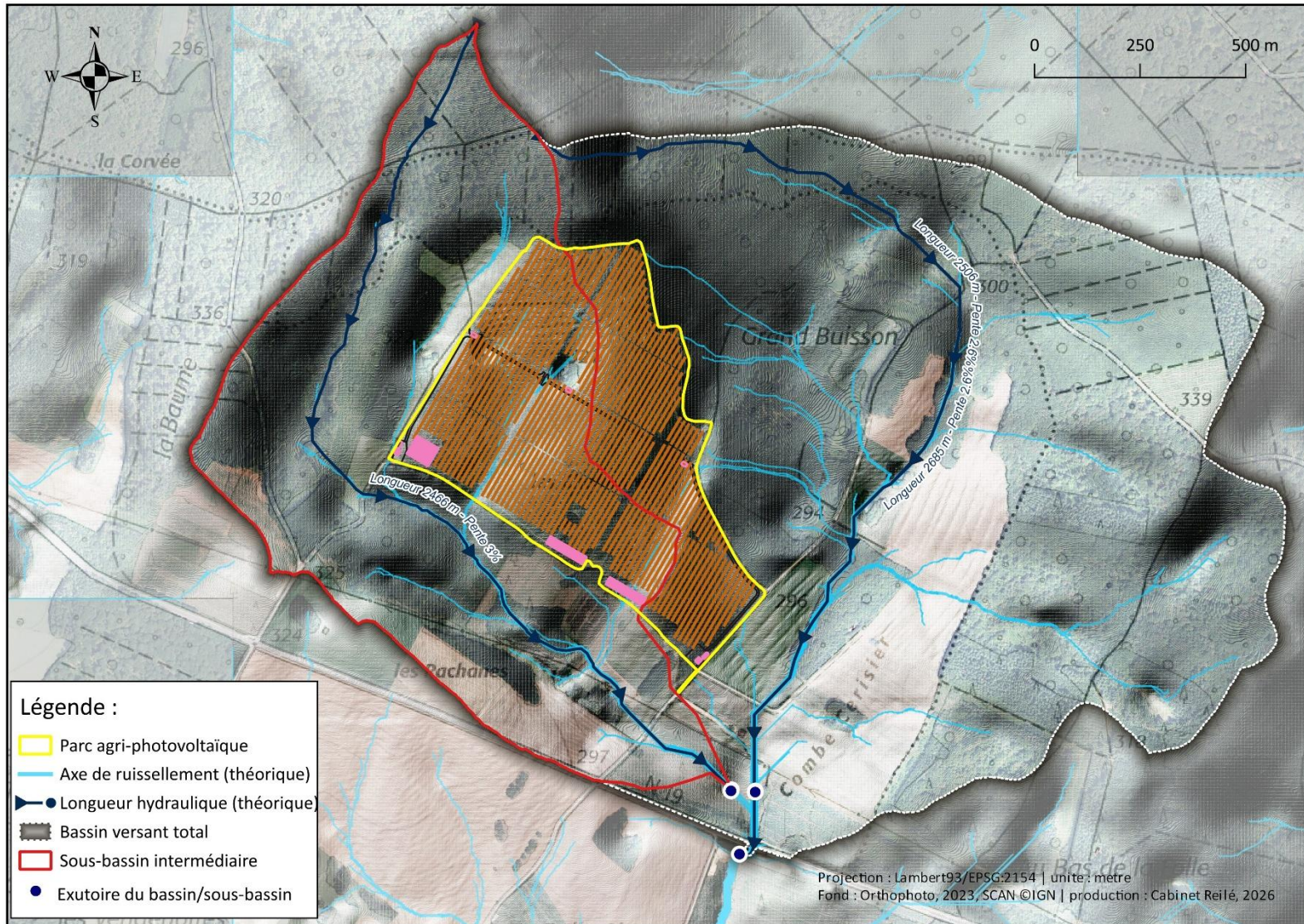
Figure 10 - Fonctionnement du bassin versant APRES aménagement.
