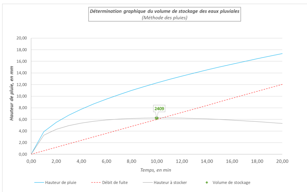
Figure 19 - Détermination du volume de stockage des eaux pluviales du sous-bassin total (BV total)
