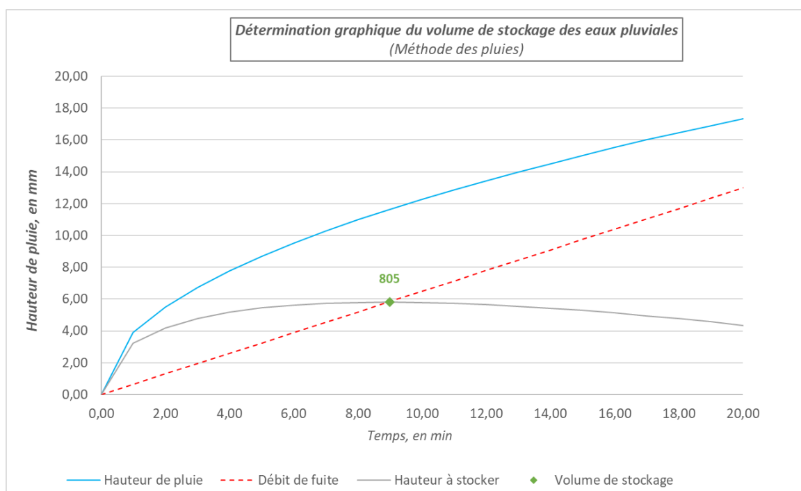
Figure 18 - Détermination du volume de stockage des eaux pluviales du sous-bassin intermédiaire (BVinter)
