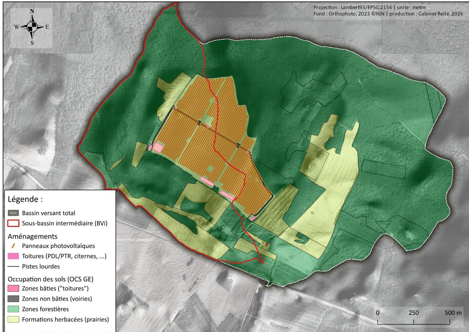
Figure 11 – Cartographie des surfaces actives du bassin versant APRES aménagement.
