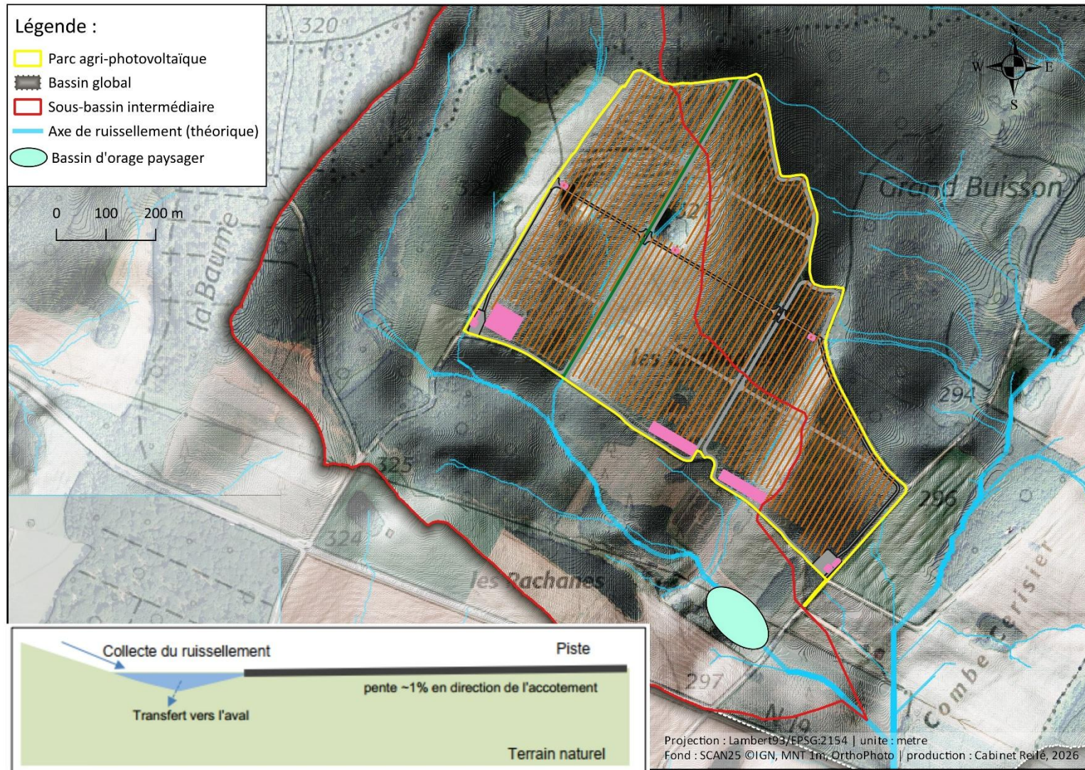
Figure 20 - Proposition d'implantation des aménagements hydraulique.
