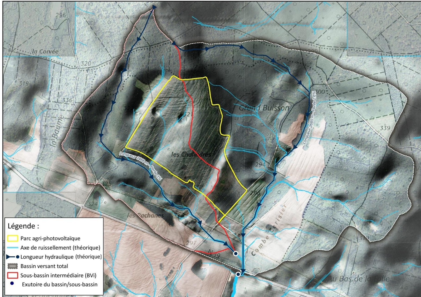
Figure 8 – Fonctionnement du bassin versant AVANT aménagement.
