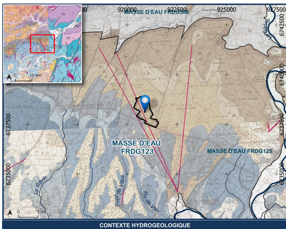
Figure 4 – Contexte géologique et hydrogéologique du projet.
