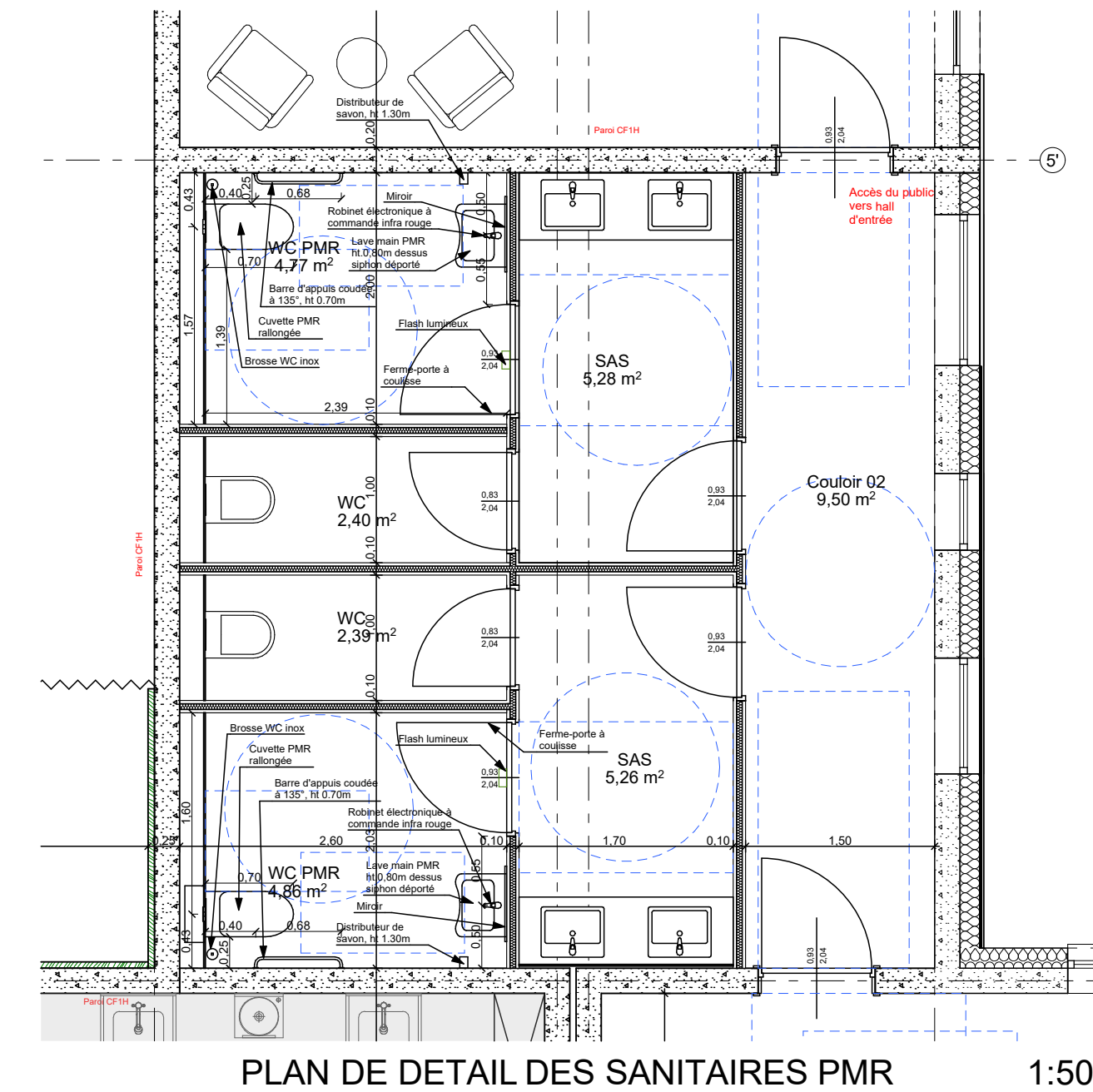
PLAN DE DETAIL DES SANITAIRES PMR 1:50
