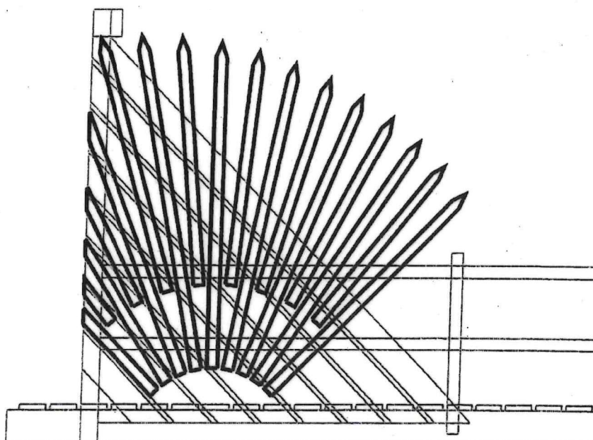
protection latérale en demi-rondins
