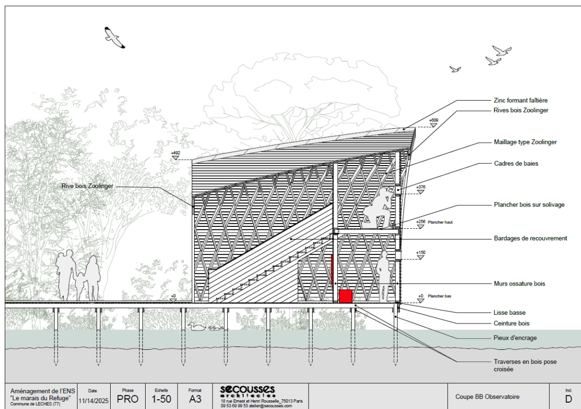
Figure 5 : Localisation et constitution de l'observatoire – PRO (SECOUSSES Architectes, 2025)
