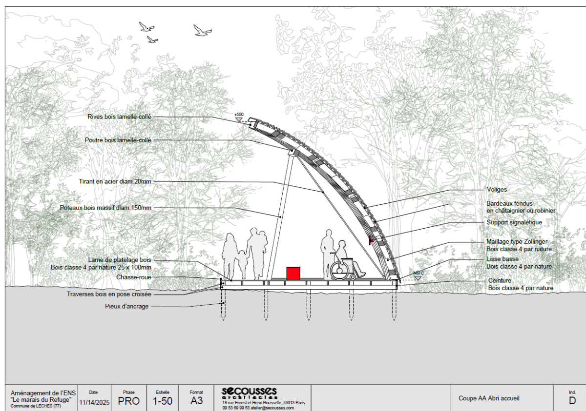
Figure 4 : Localisation et constitution de la structure de l'abri d'accueil – PRO (SECOURSSES Architectes, 2025)
