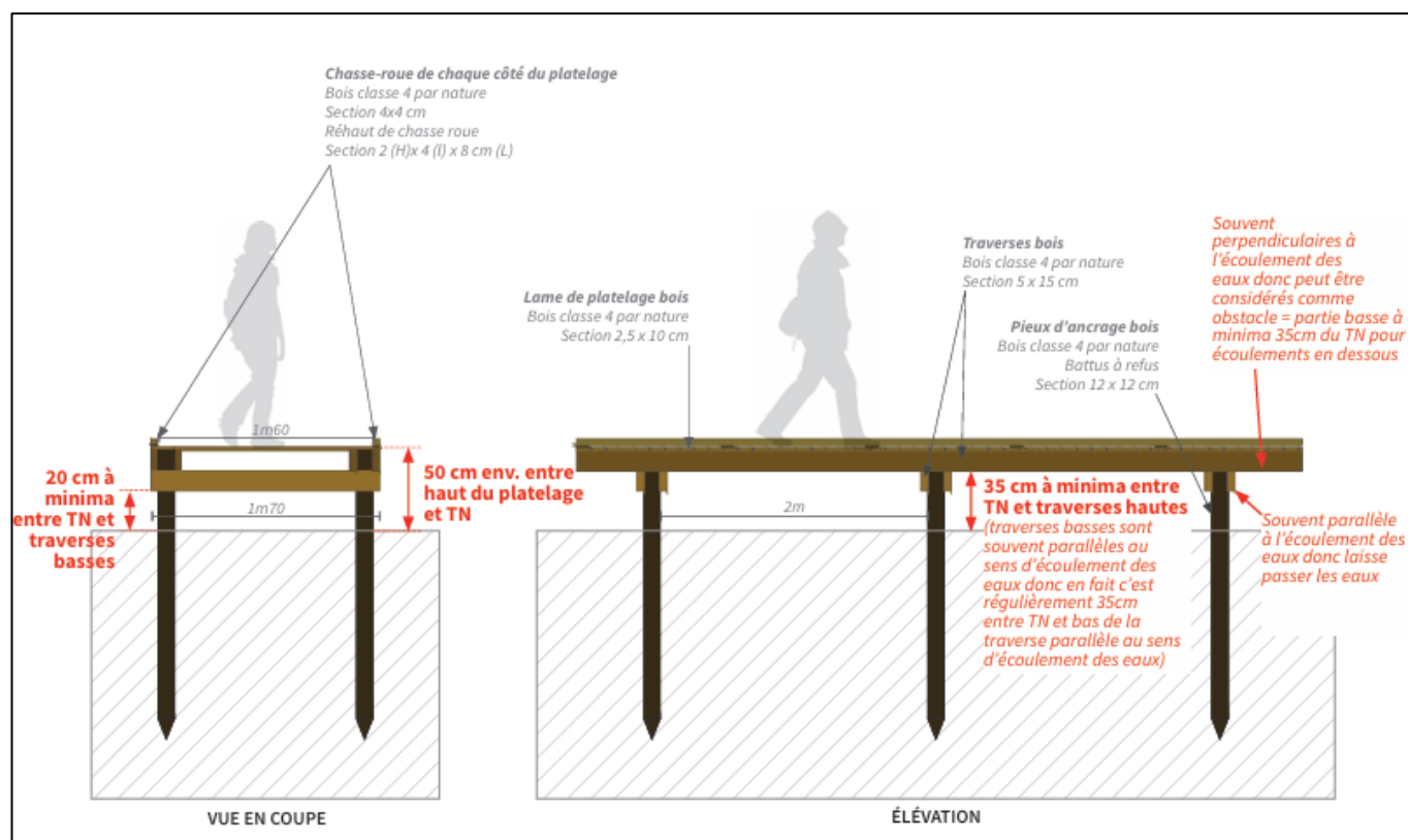
Figure 2 : Platelage bois : vues en coupe - PRO (Atelier-Kosmes, 2025)
