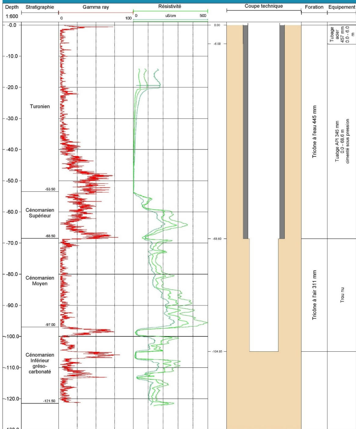
Figure n°4 : Coupes technique, stratigraphique et diagraphies du forage de Romegoux « Les Groies de Bertin F 2 »
