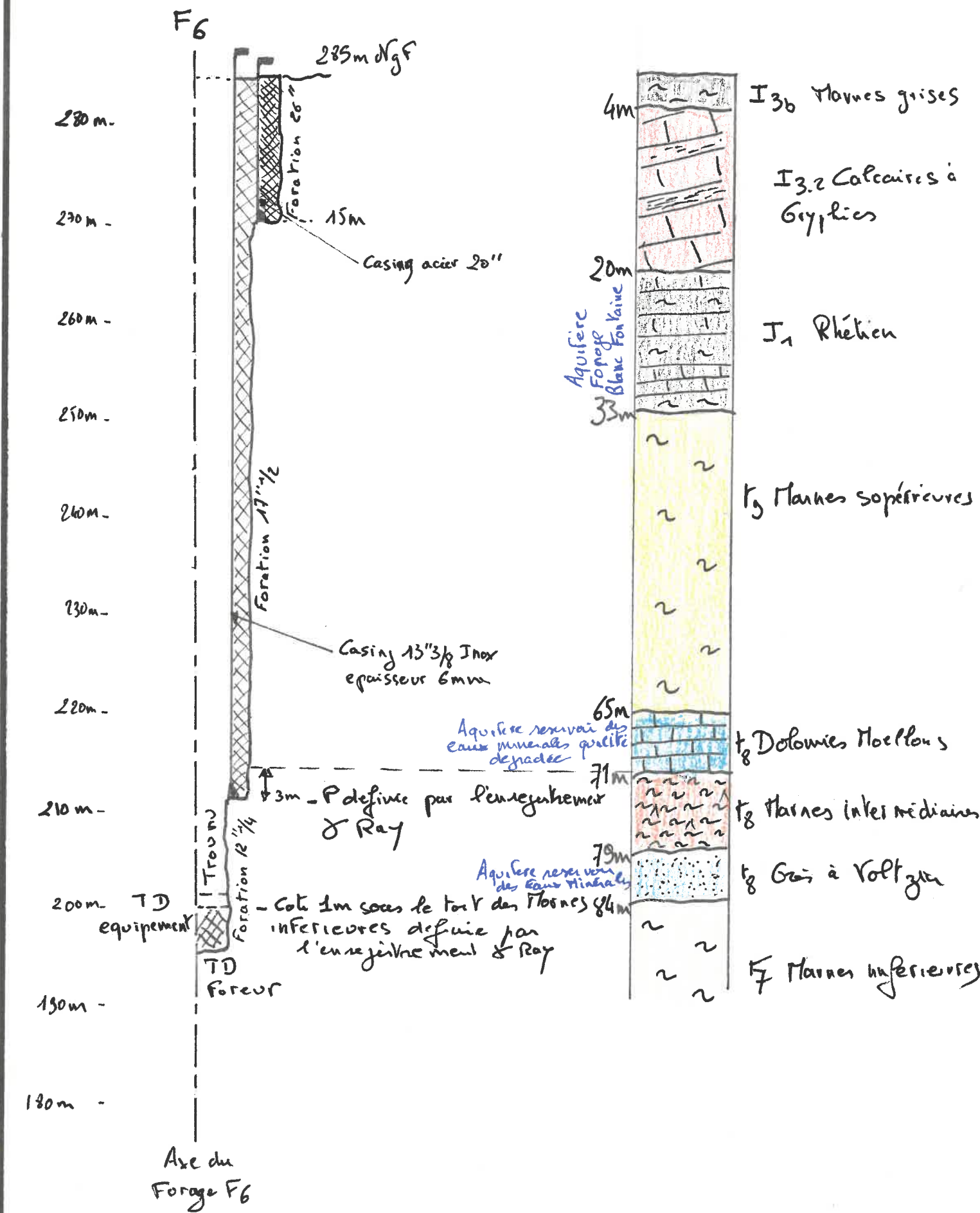
LES EAUX MINÉRALES DE VÉLIEMINFRÖY DOSSIER DE DÉCLARATION DES TRAVAUX DE FORAGE DE RECONNAISSANCE F5 & F6 Illustration N°7 : Coupes techniques prévisionnelles et géologiques du Forage F6
