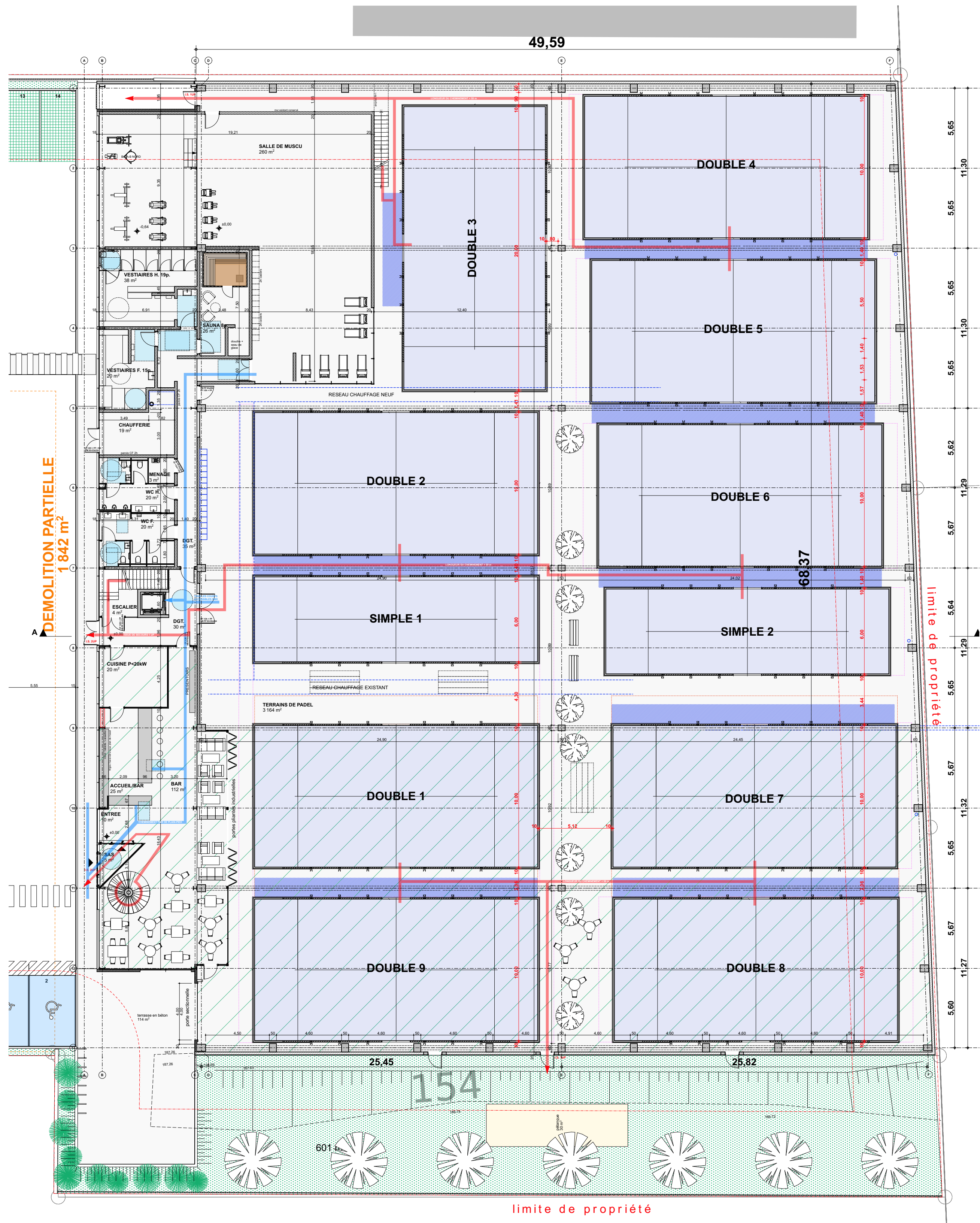
PLAN DU REZ-DE-CHAUSSEE
