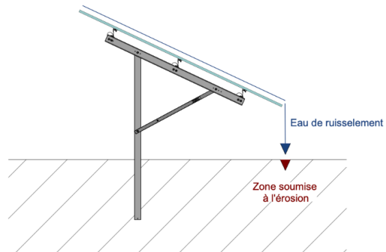
Cas n°1 : Structures supportant des panneaux joints les uns les autres ( non concerné par le projet )
