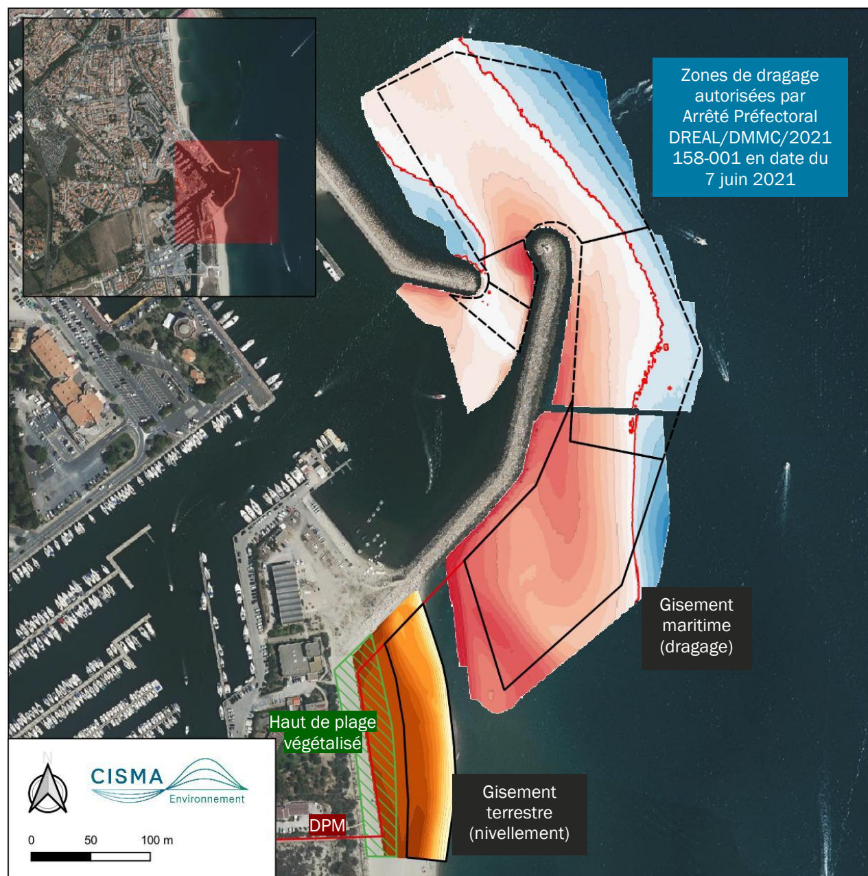
Figure 1 : Nouvelles zones à draguer (en mer) et à niveler (sur la plage) (fond : bathymétrie avril et septembre 2025, CISMA Environnement, d'après GEO CART'EAU ; topographie février 2026, CISMA Environnement)
