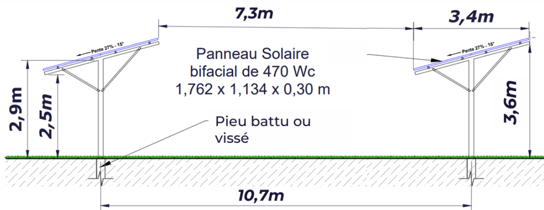
Plan de détail des tables photovoltaïques
