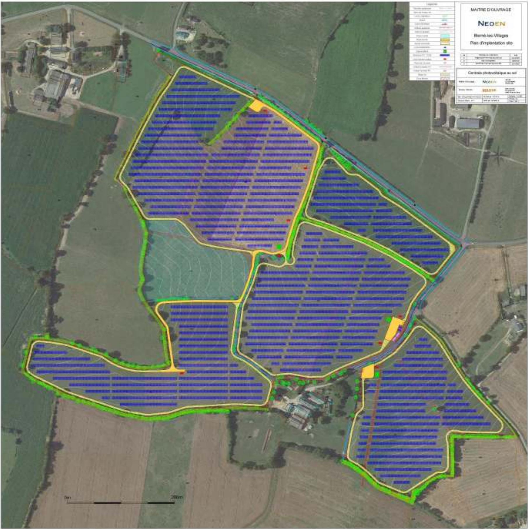
Figure 101 : Plan de masse du projet (08/10/2025)
