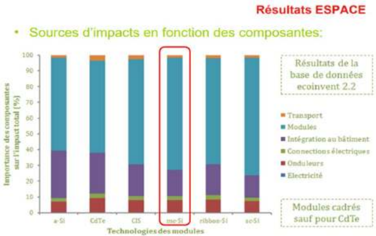
Figure 104 : Sources d'impact d'un projet PV
