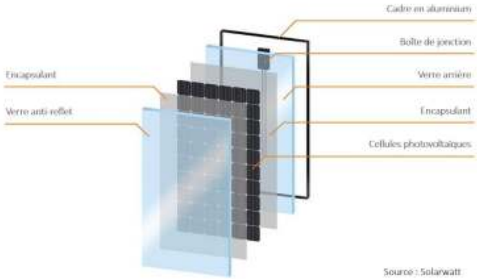
Figure 97 : Décomposition d'un module photovoltaïque
