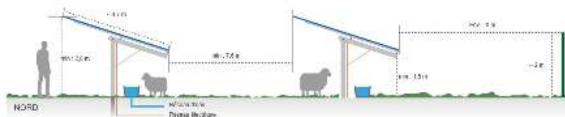
Figure 98 : Schéma d'une installation agrivoltaïque ovine
