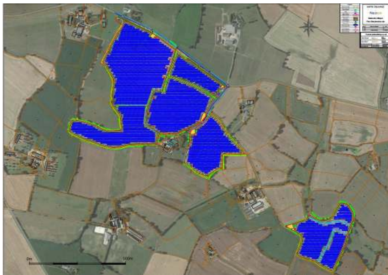
Figure 93 : Scénario d'implantation n°1
