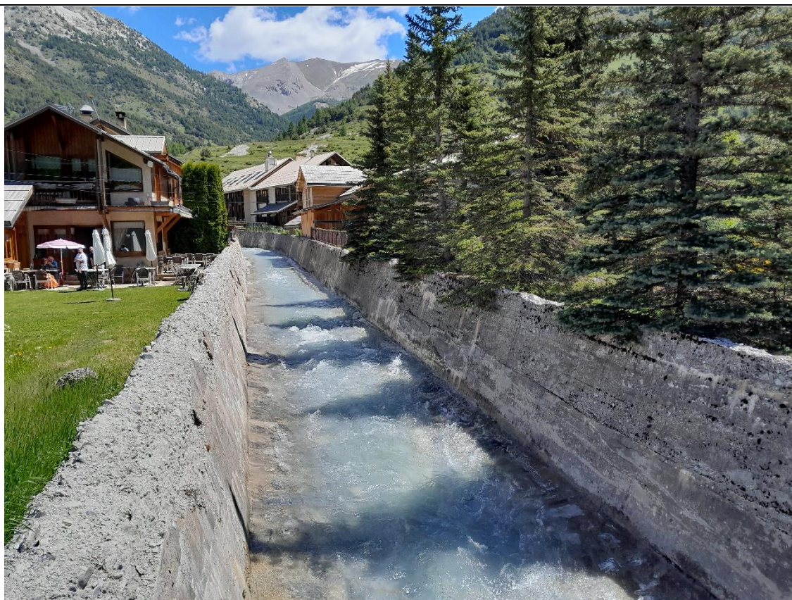
↑ Fig. 5 Chenal dans le bourg, vue vers l'amont. Etat des sommets de digues (rive droite)
