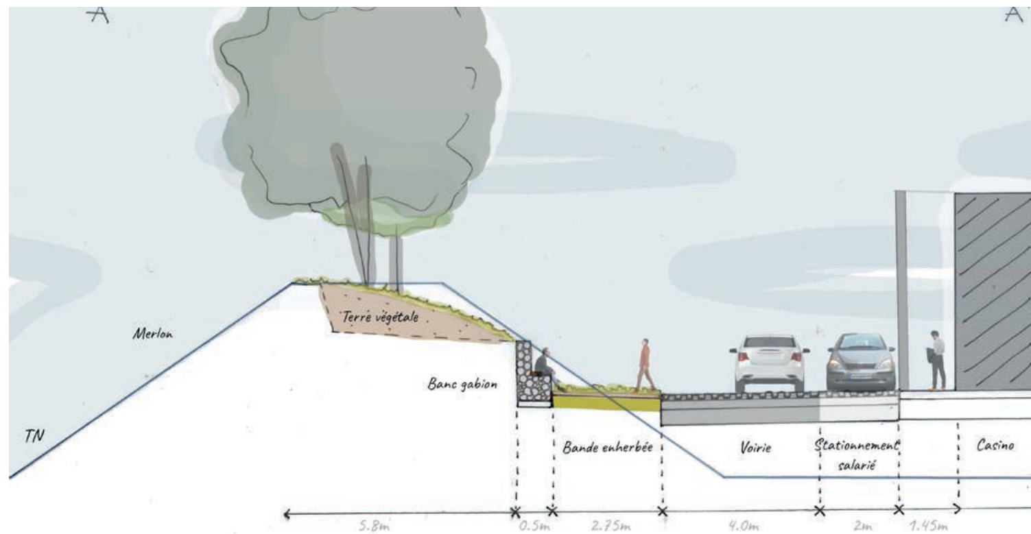
Coupe de principe d'aménagement du merlon au nord du Casino
