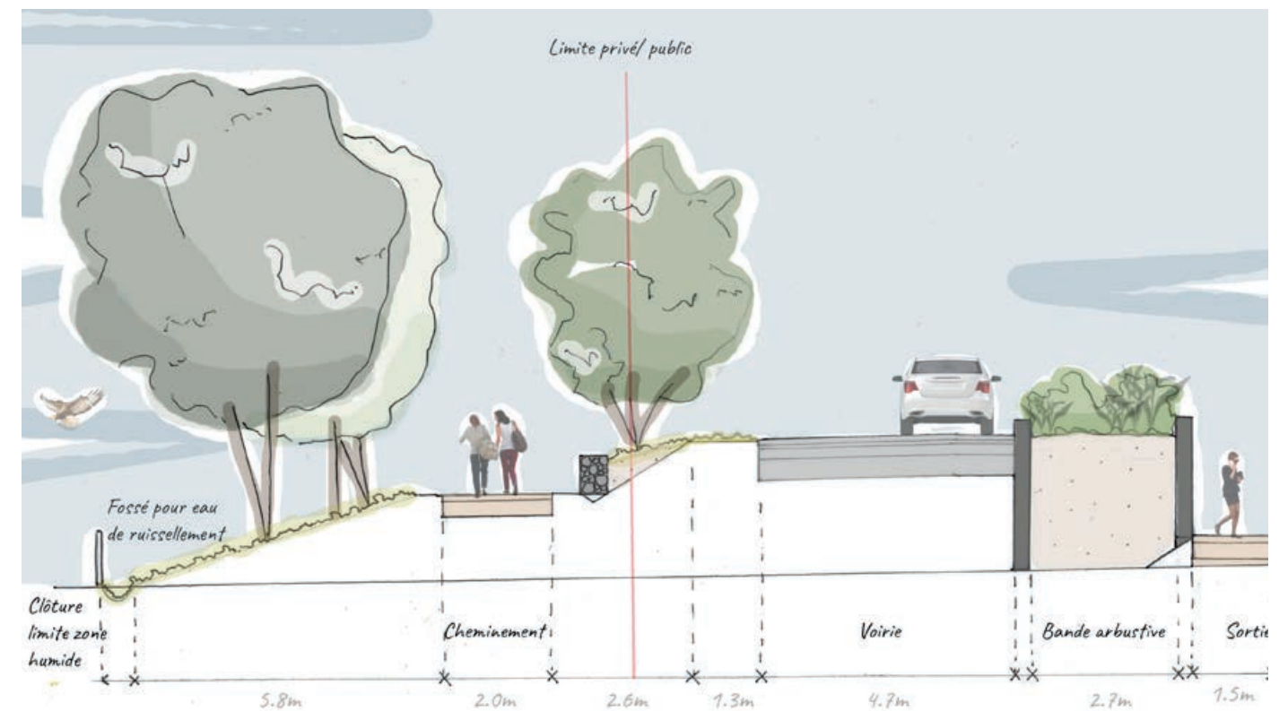
Coupe de principe d'aménagement de la voie d'accès au Casino côté zone humide
