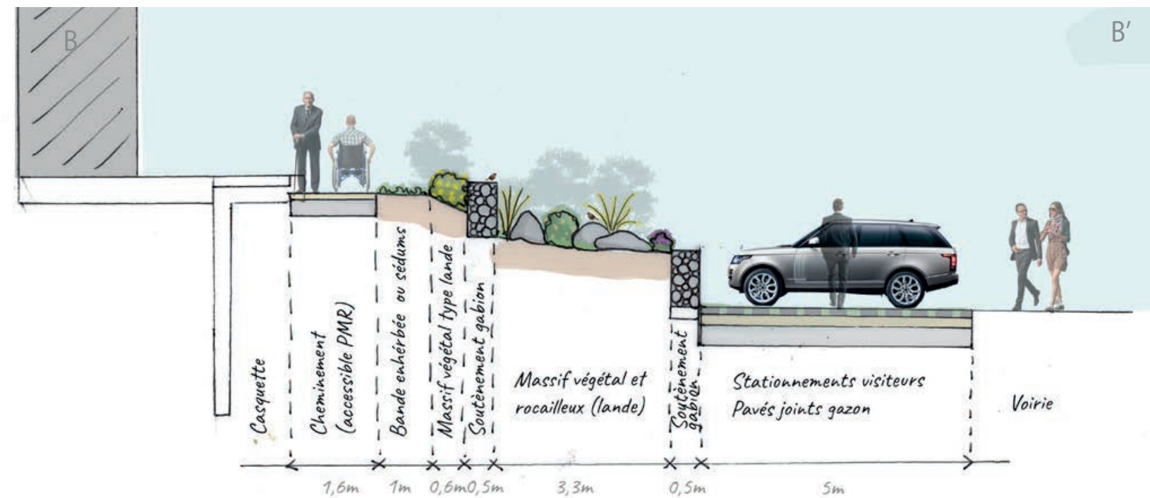
Coupe de principe d'aménagement des terrasses de landes fleuries devant le Casino
