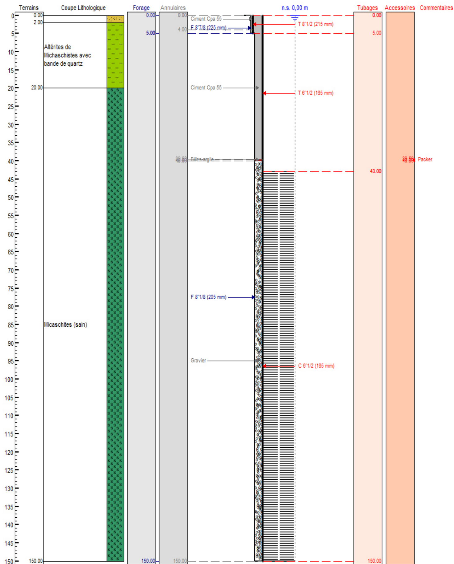
Coupe prévisionnelle du forage
