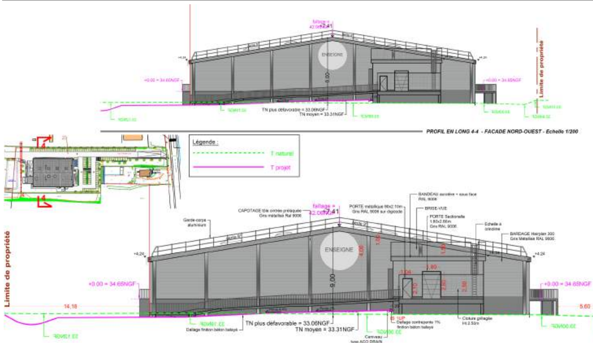
Figure 9 : Profils en long – Façade Nord-Ouest
