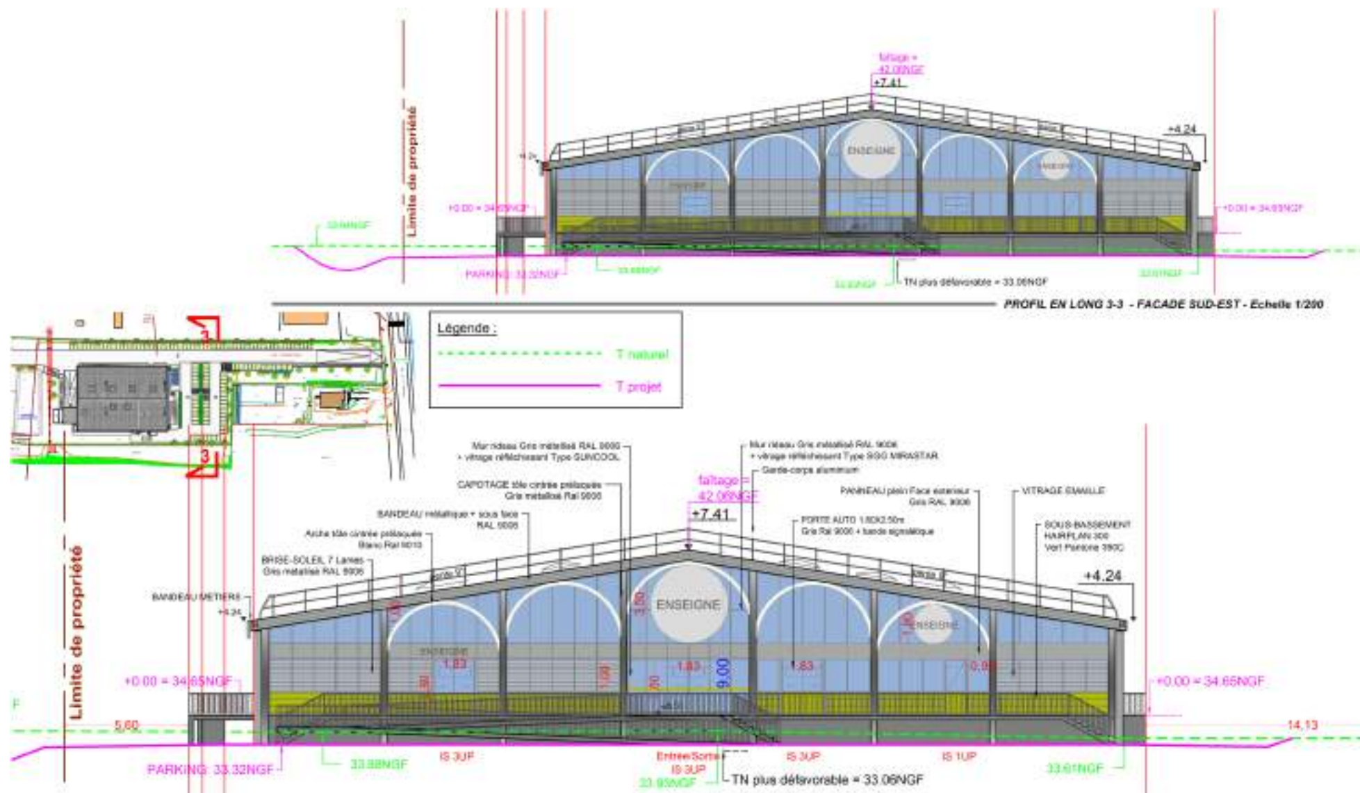
Figure 8 : Profils en long – Façade Sud-Est
