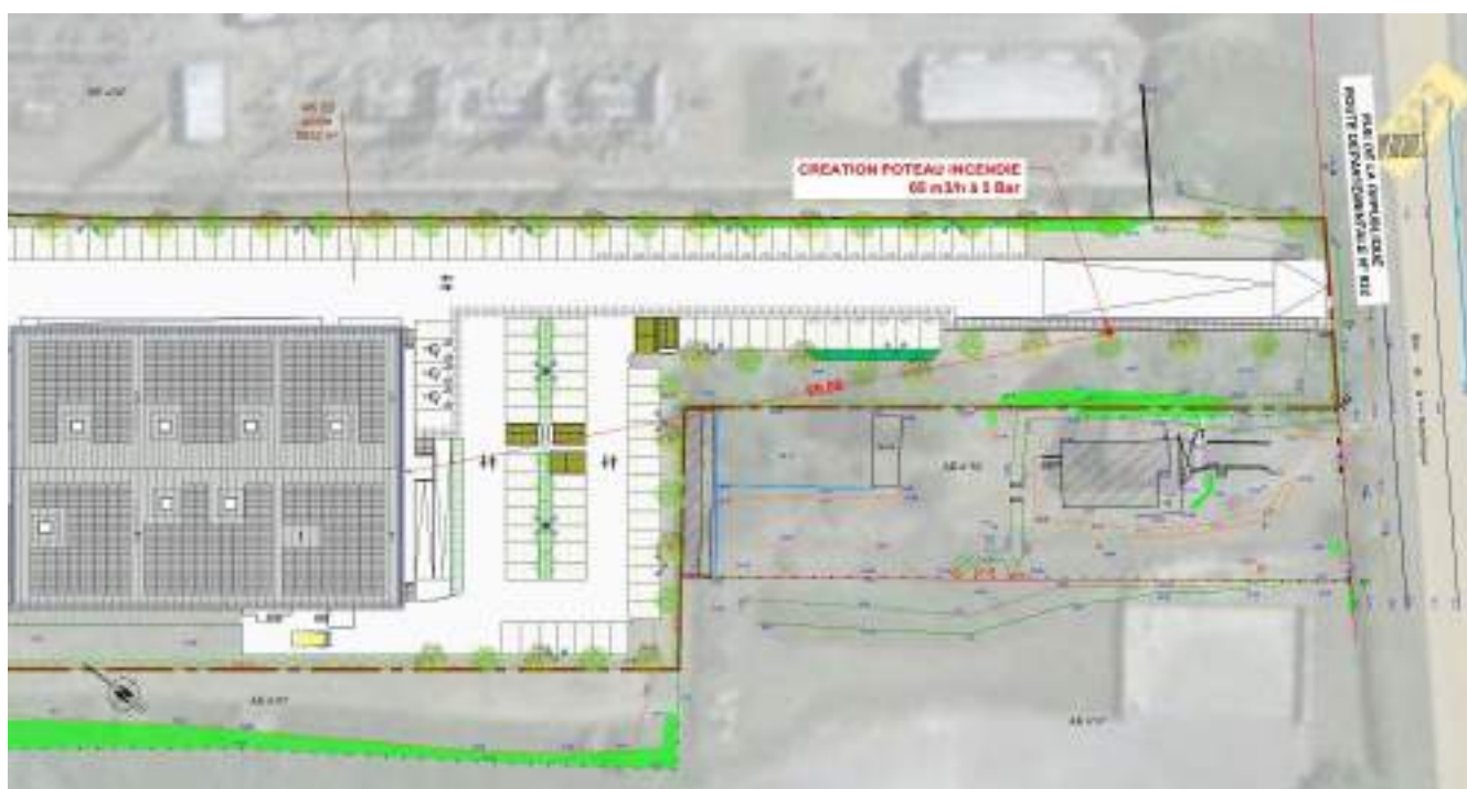
Figure 10 : Localisation du poteau incendie à créer
