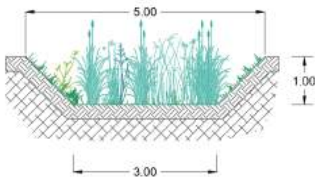
Figure 11 : Coupe d'une noue avec plantes macrophytes
