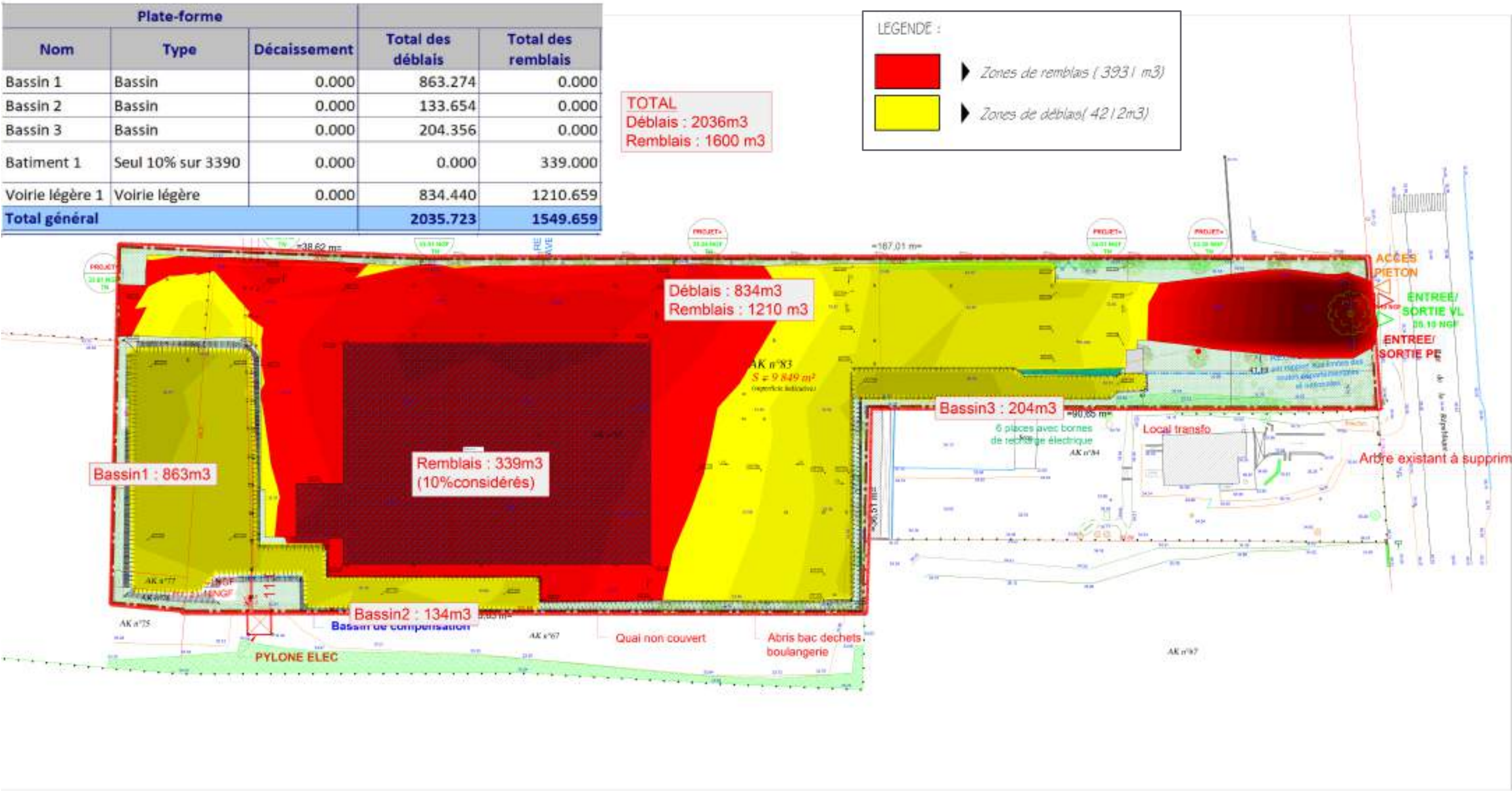
Figure 14 : Plan de compensation des eaux – Décembre 2025
