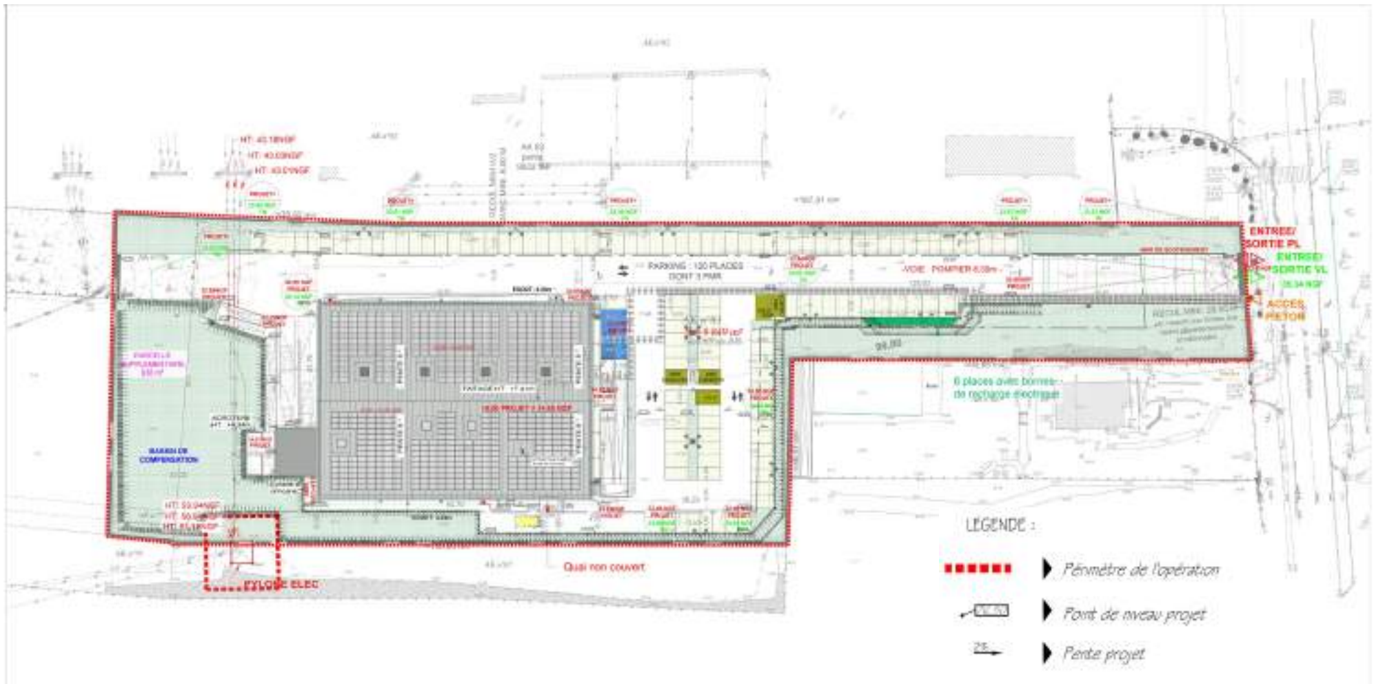
Figure 18 : Plan de nivellement du site – Juillet 2025
