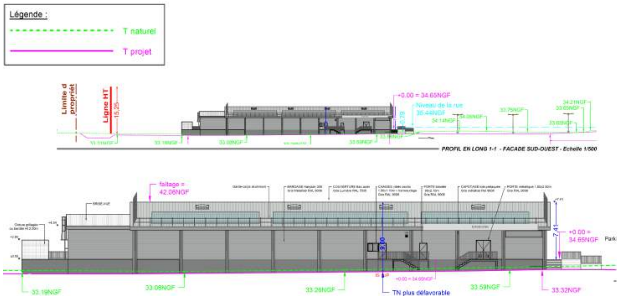
Figure 6 : Profils en long – Façade Sud-Ouest
