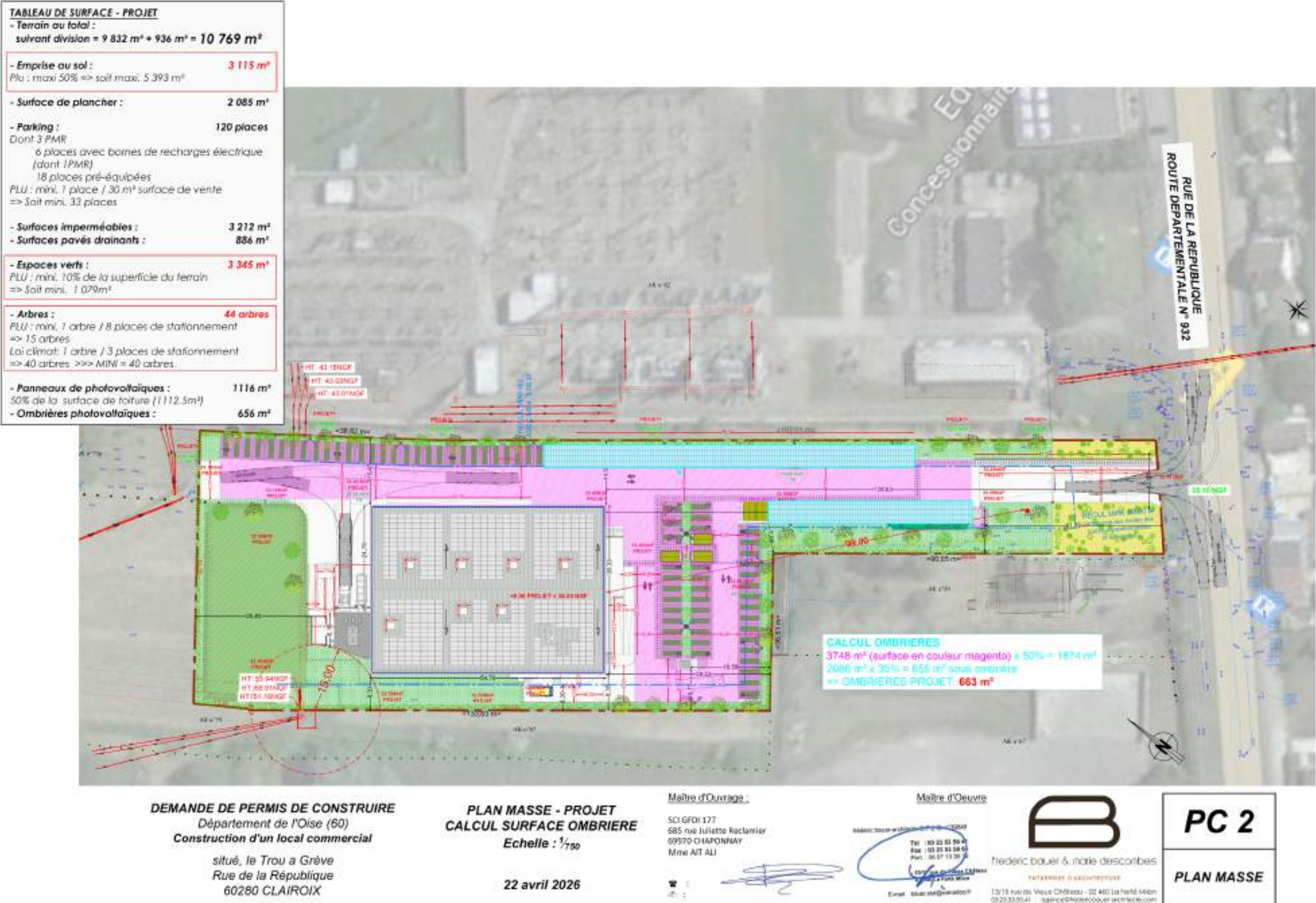
Figure 5 : Plan masse du projet – Avril 2026
