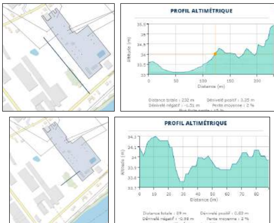
Figure 17 : Topographie et Profils altimétriques (A-B et C-D) du terrain
