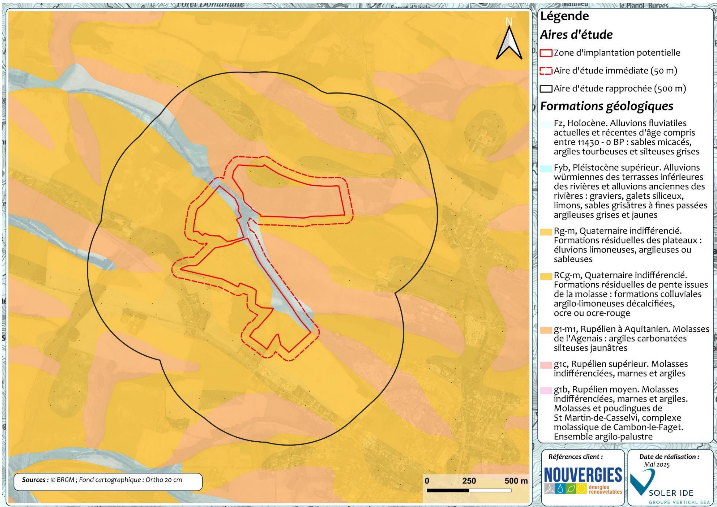
Figure 27 : Carte géologique au sein et à proximité de l'aire d'étude immédiate
