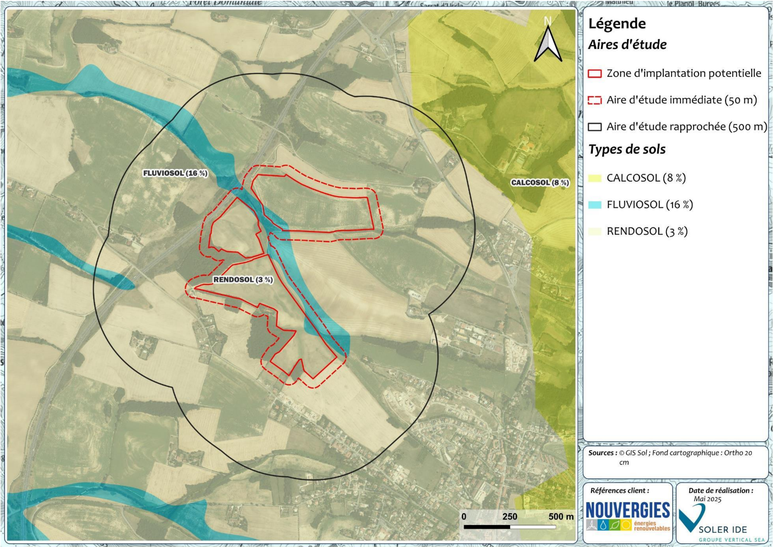
Figure 26 : Cartographie des sols sur et à proximité de l'aire d'étude immédiate
