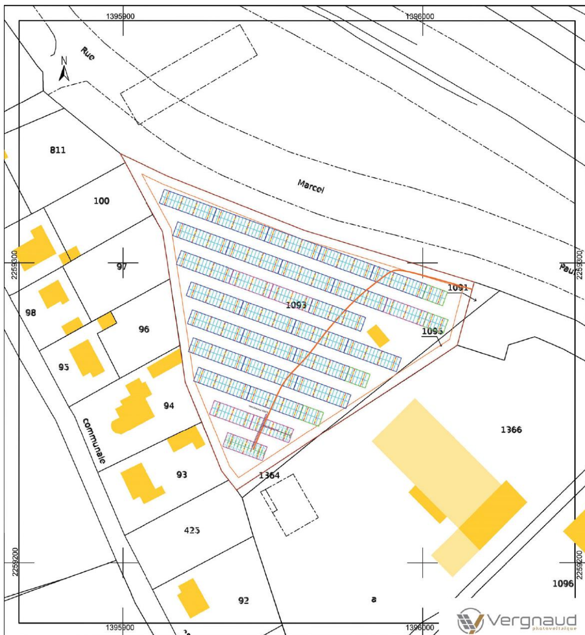
Figure 1 : Projet initial
