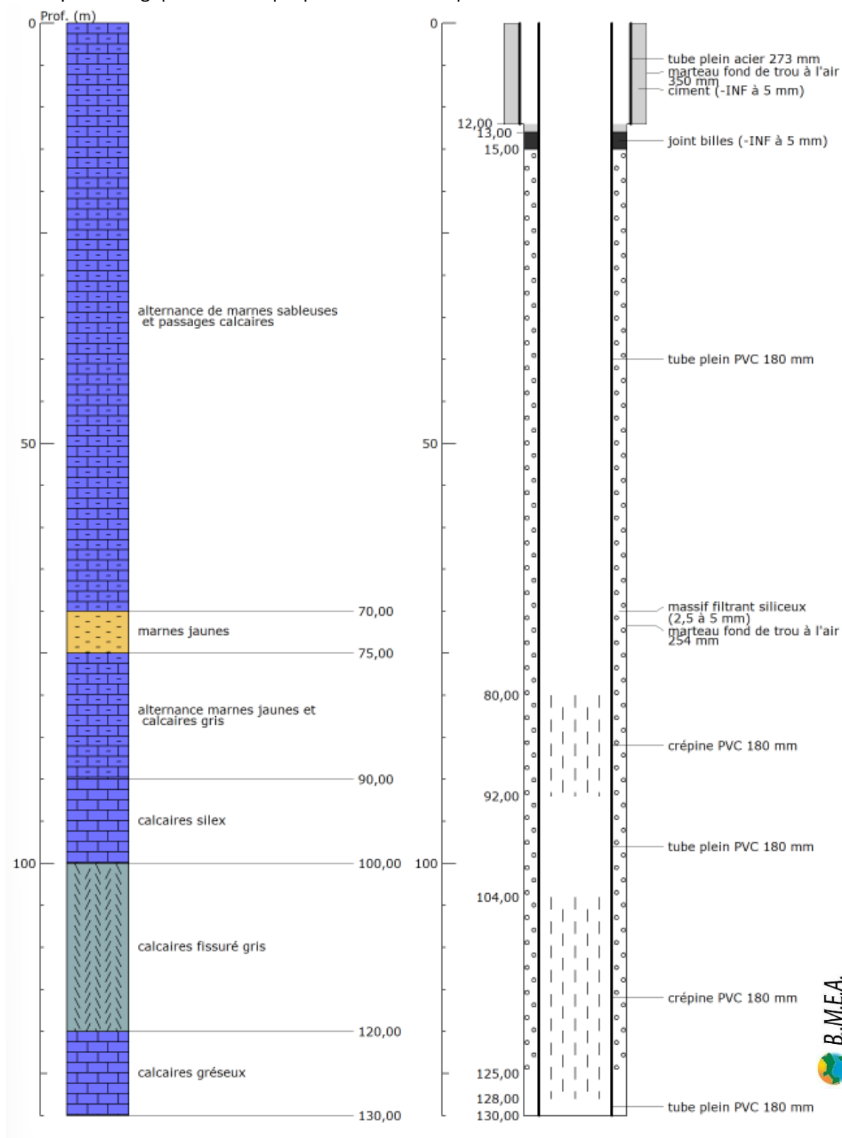
Pièce graphique n° 4 : Coupe lithologique et technique du forage projeté
