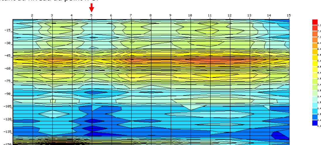
Pièce graphique 11 : Profils d'imagerie électrique n° 3 de la commune de CAVES
