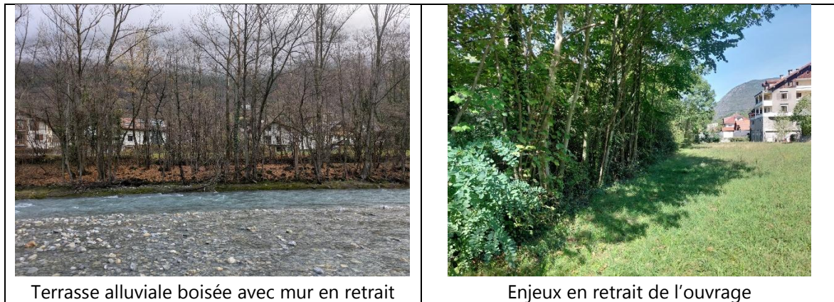
Figure 2 : Photographies du tronçon 1 de la digue du plan du Truy
