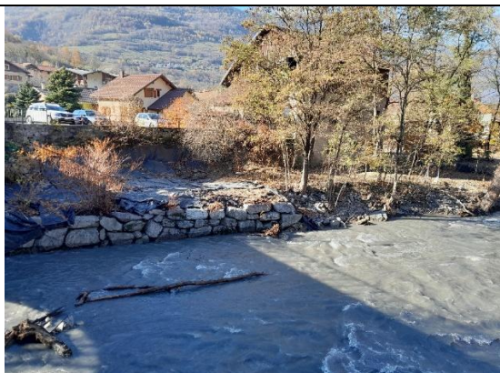
Soutènement à l'approche du pont
