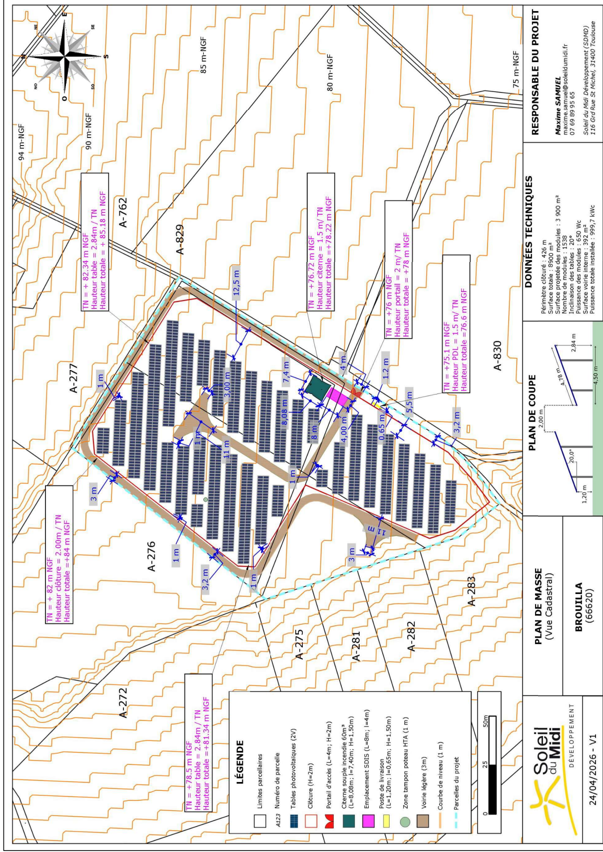
Figure 14 : Plan de masse sur vue cadastrale
