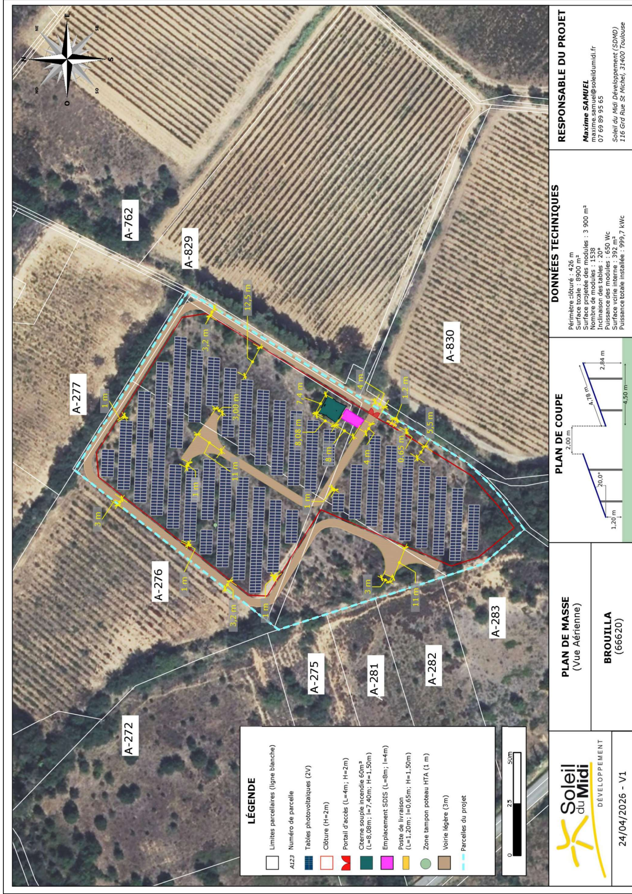
Figure 15 : Plan de masse, vue aérienne
