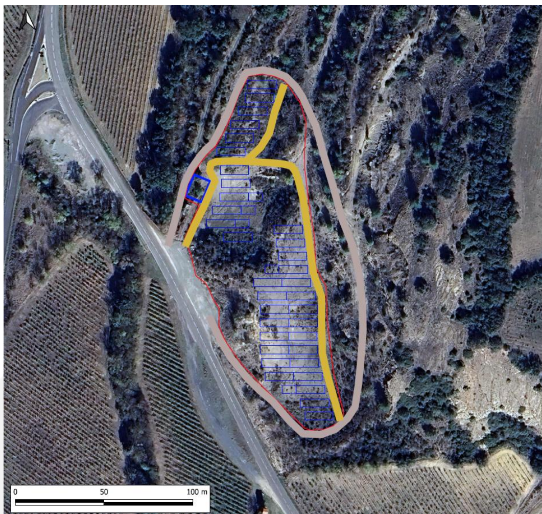
Plan à l'échelle cadastrale
