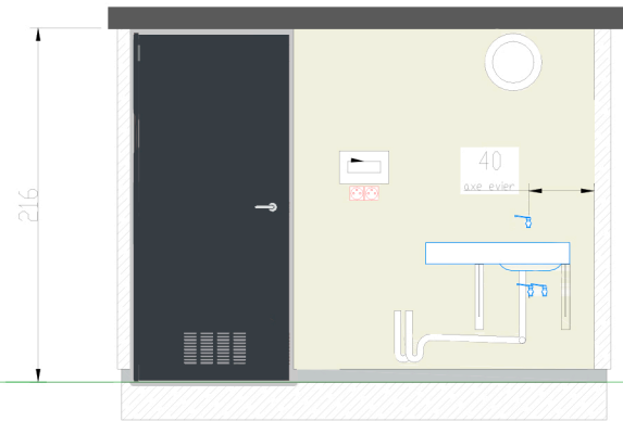
COUPE C-C (Vue intérieur des buanderies)
