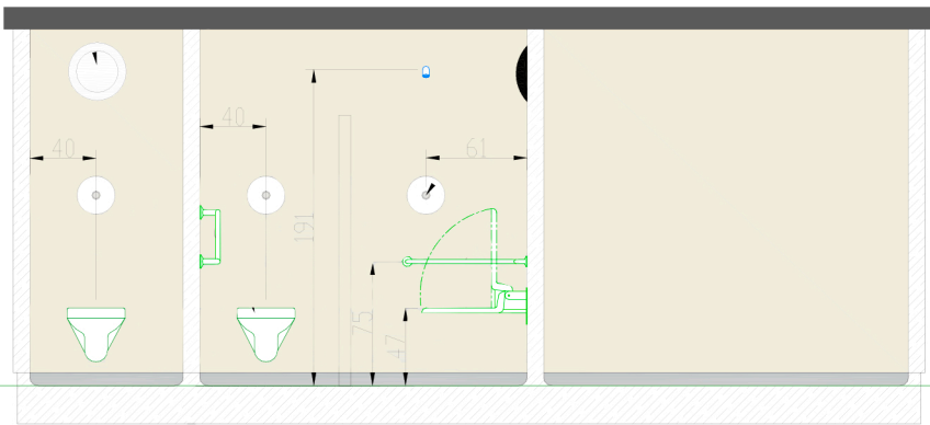
COUPE A-A (vue intérieur cabines)
