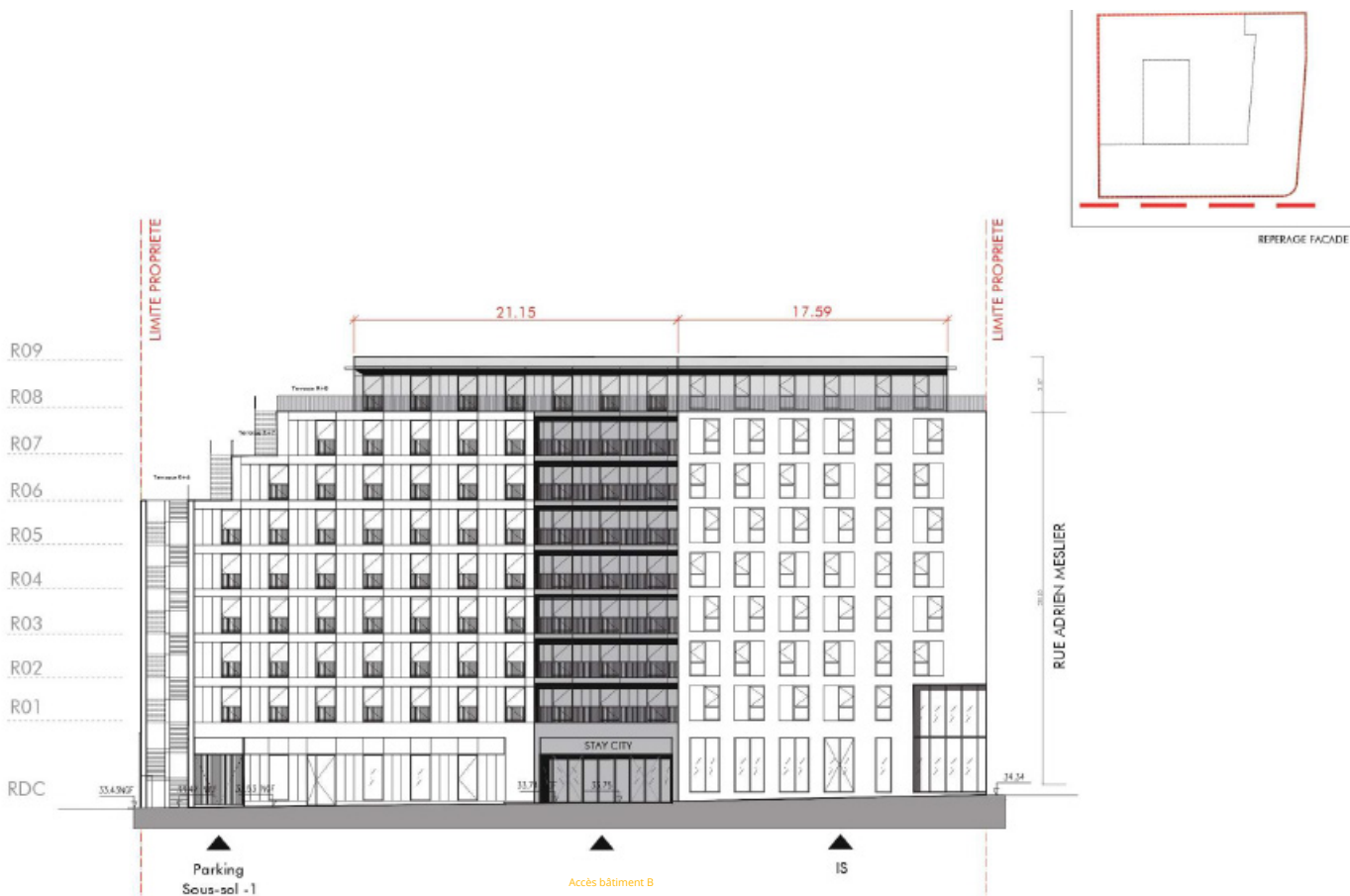
Fig.53 : Façade rue Paulin Talabot (CALQ, 2026)
