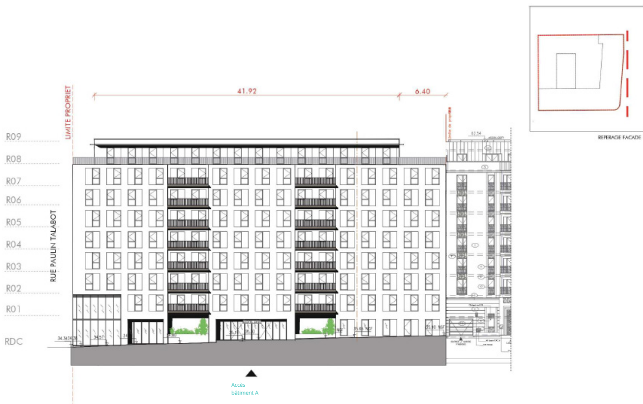
Fig.52 : Façade rue Adrien Meslier (CALQ, 2026)
