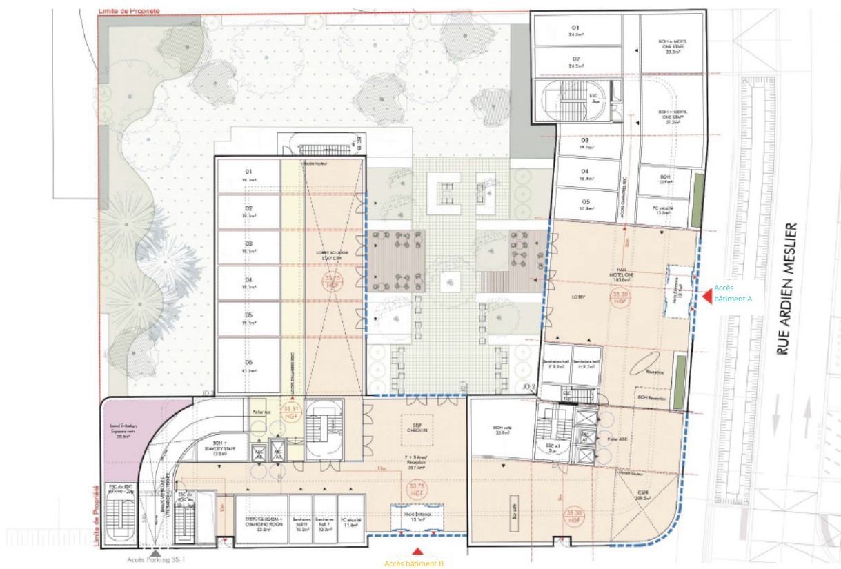
Fig.51 : Plan rez-de-chaussée (CALQ, 2026)
