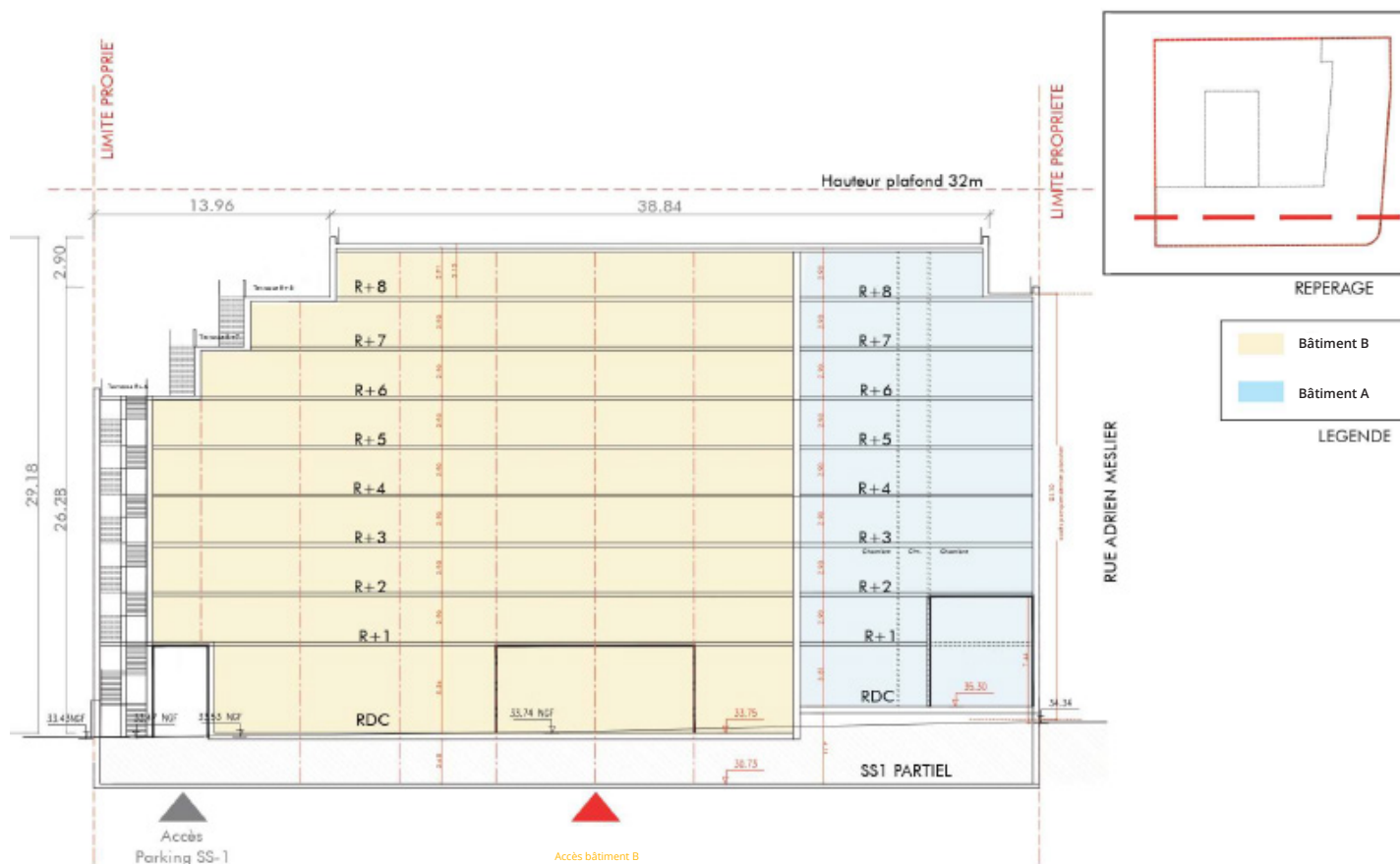
Fig.57 : Coupe BB' (CALQ, 2026)
