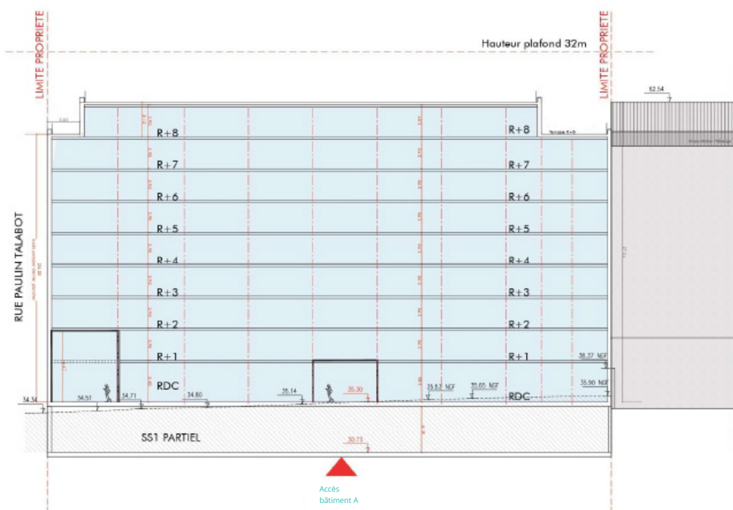
Fig. 54 : Coupe AA' (CALQ, 2026)
