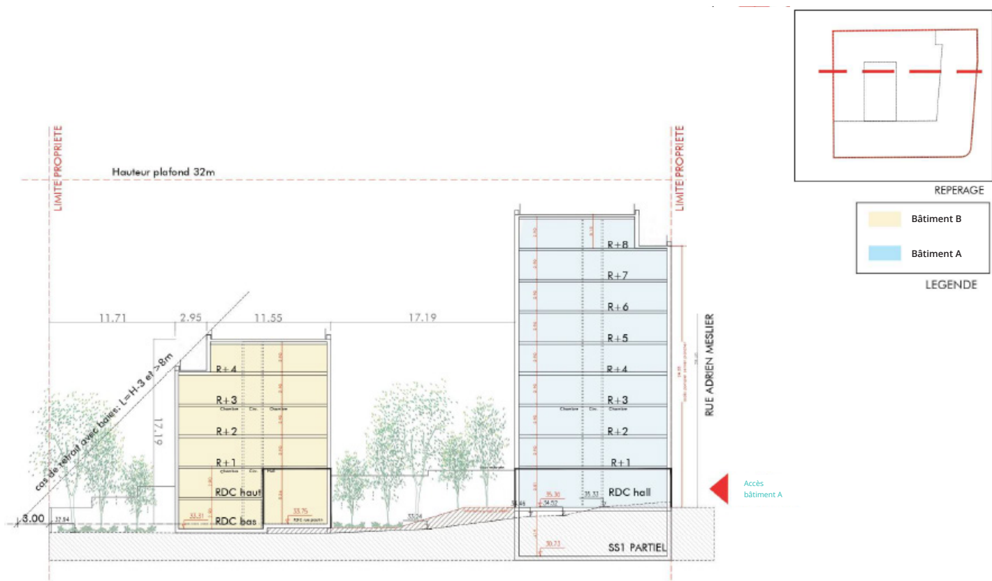
Fig.56 : Coupe CC' (CALQ, 2026)
