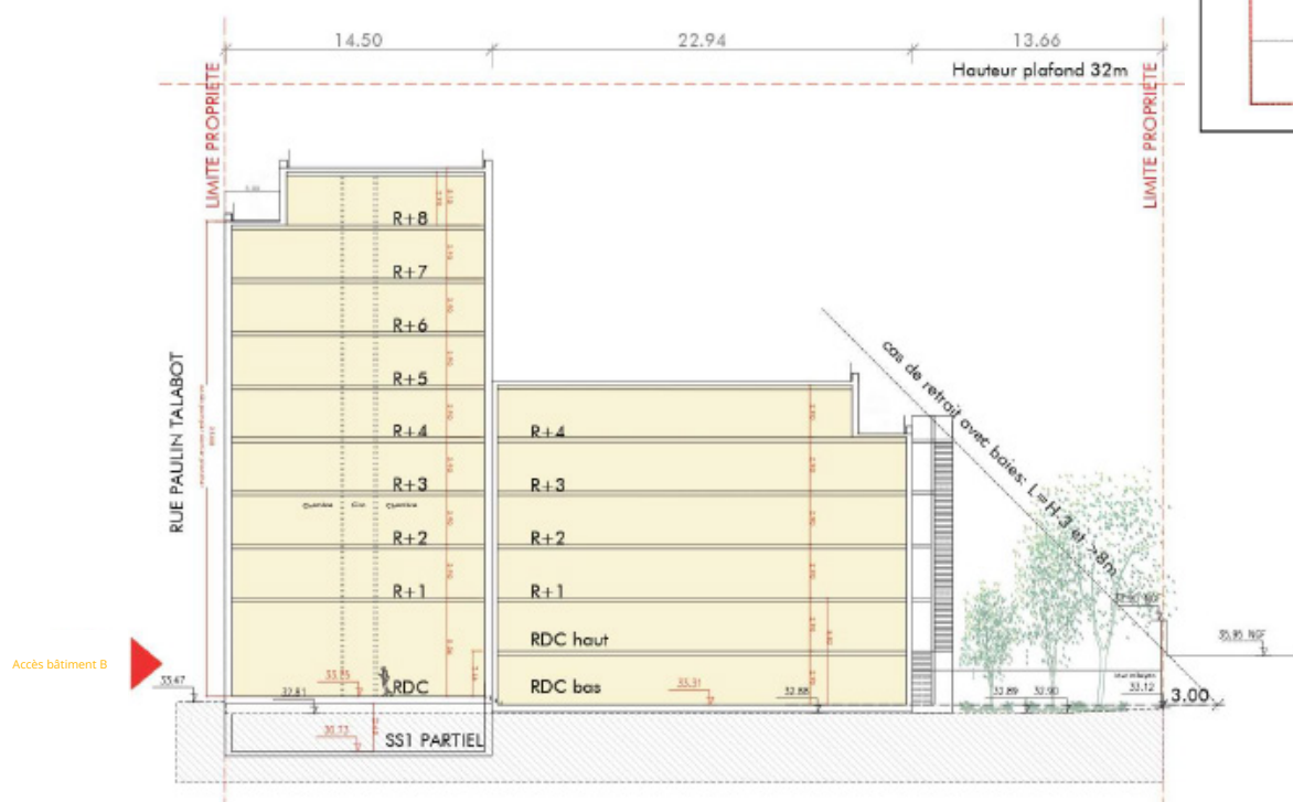
Fig. 55 : Coupe BB' (CALQ, 2026)
