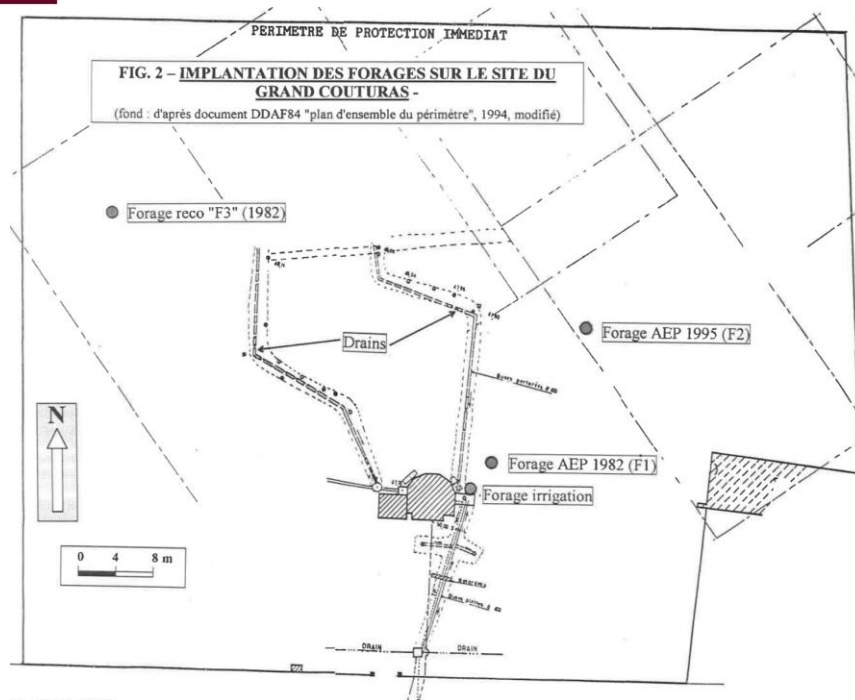
Figure 5 : Plan du site et du périmètre de protection immédiate (Mallessard , 2001)
