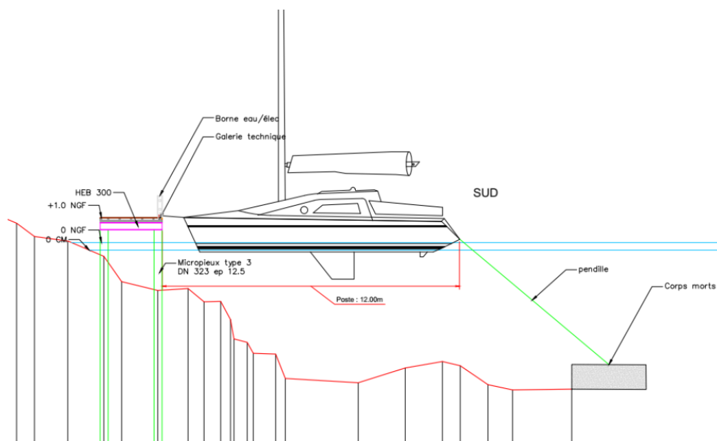
Structure type du ponton
