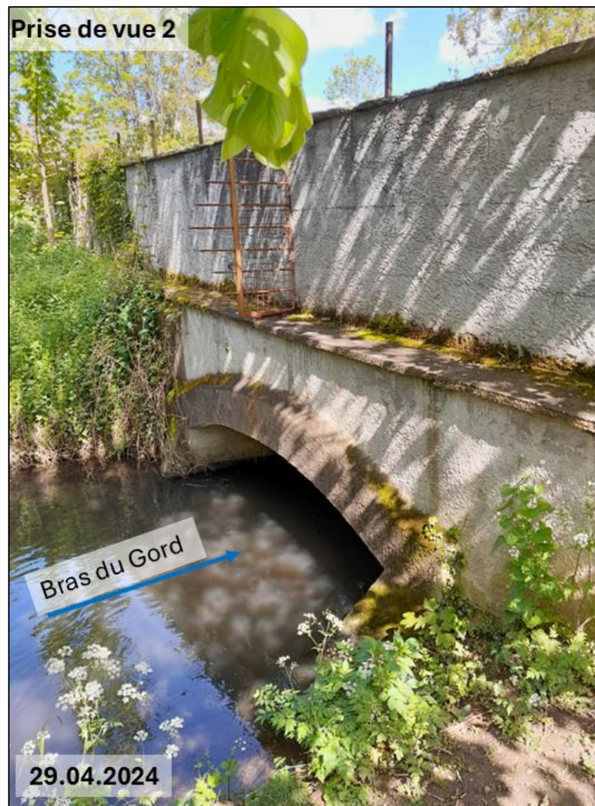
Figure 5 : Photographie n°2 – Vue de l'aval du tronçon 2 et amont du pont de la rue du Domaine
