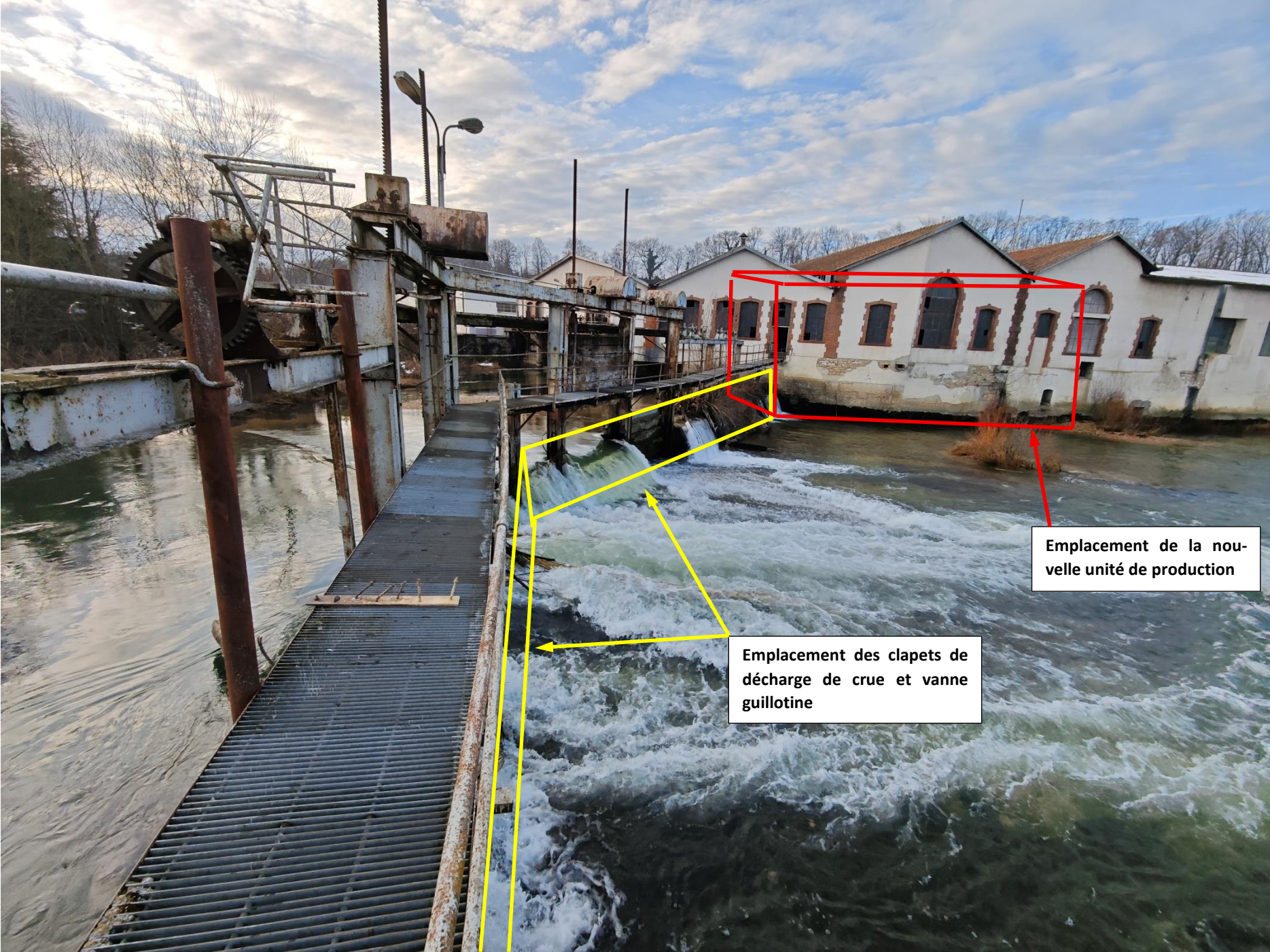
Vue rive gauche
