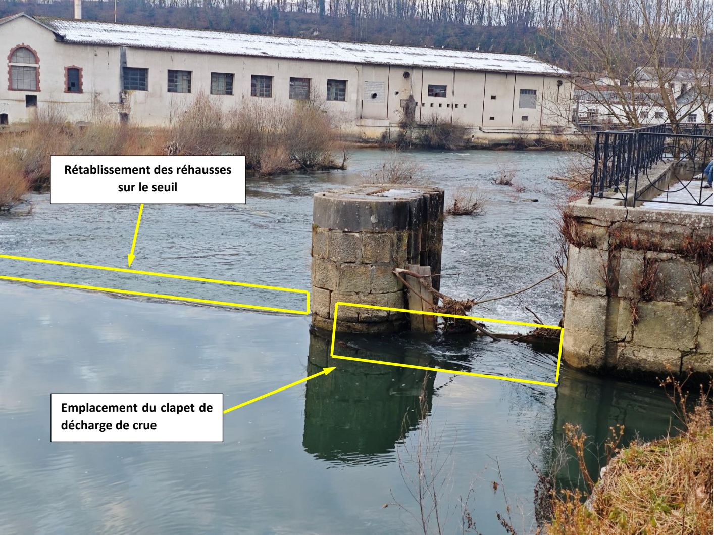
Vue rive droite
