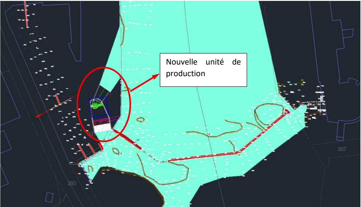
Implantation et dimensions (Vue de dessus)
