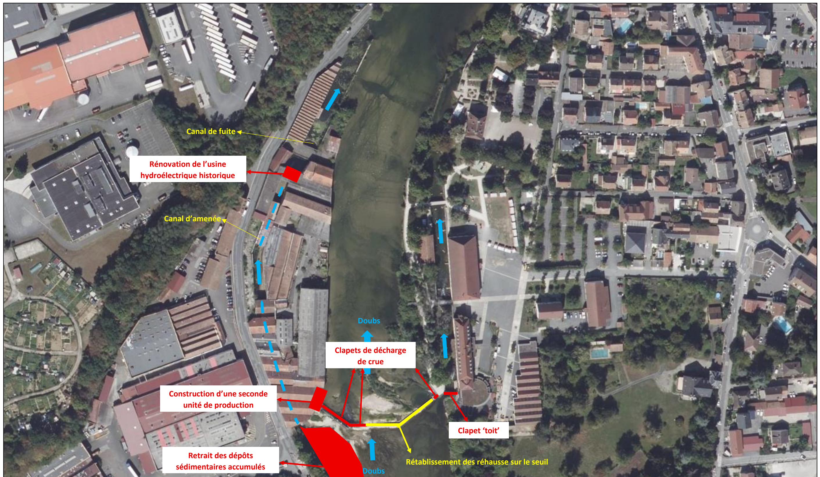
Figure 2 : Présentation synthétique du projet (vue aérienne)
