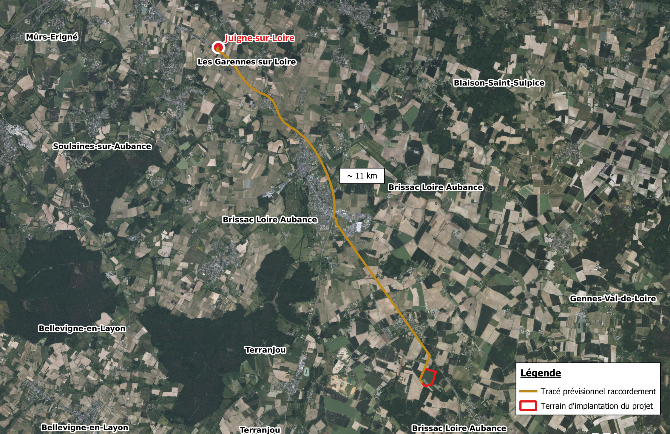
Carte du tracé prévisionnel du raccordement au poste source
