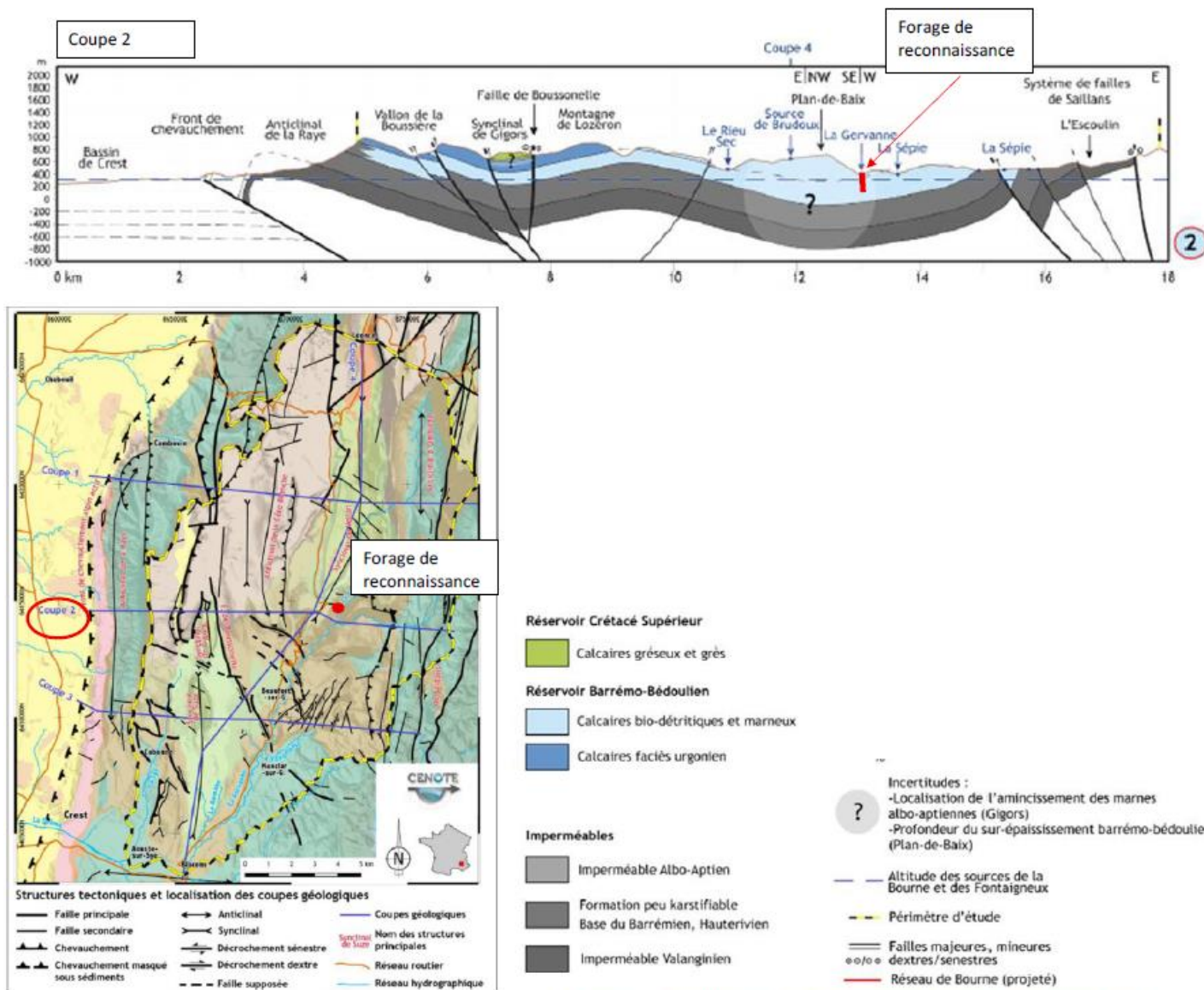
Figure 3 : Carte géologique du secteur et coupe géologique (extrait rapport Antea)
