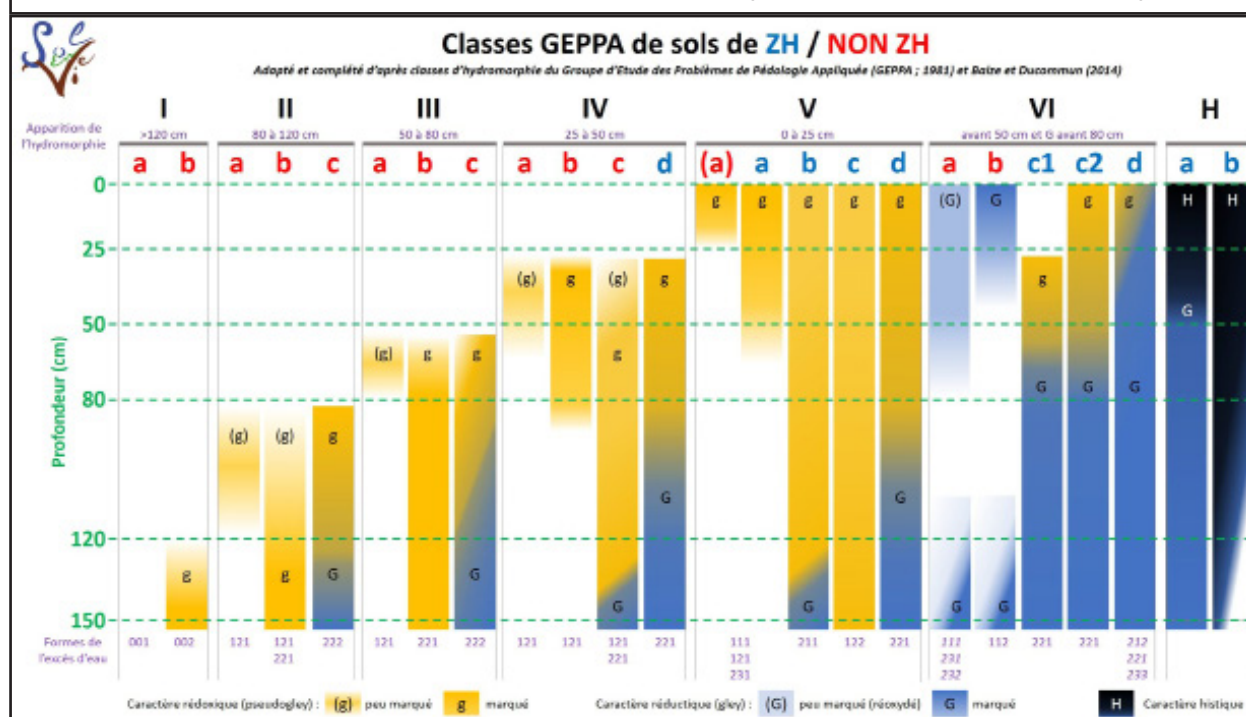
FIGURE 9 : CLASSE D'HYDROMORPHIE (GEPPA, 1981, MODIFIÉ)
