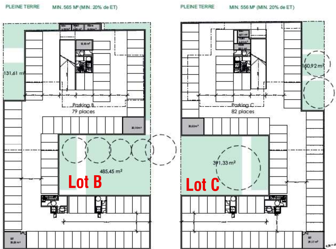
Figure 12 : Plan du souterrain et taux de pleine terre des lots B et C (Etude Architecturale, Atelier Martel)
