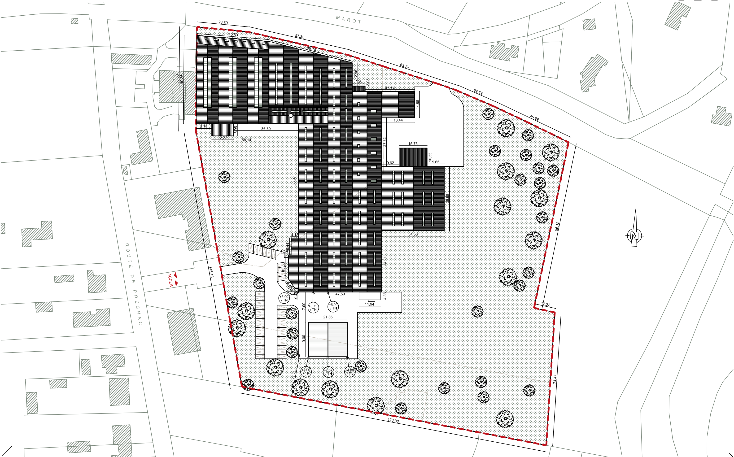
PLAN DE MASSE TOITURE PROJET
