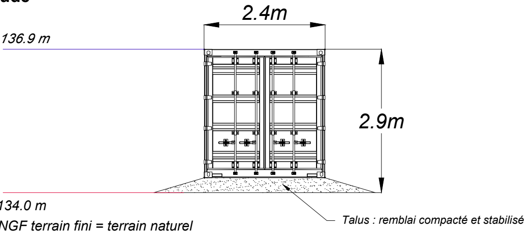
FACE EST
