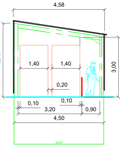
Coupe sur transfert chariot autonome type agv
