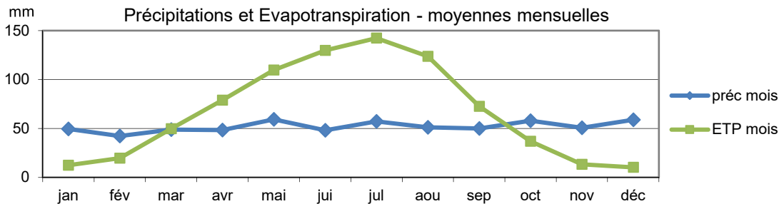
Figure 34. Précipitations et Evapotranspiration, station de Brétigny sur Orge, 1981-2010.
