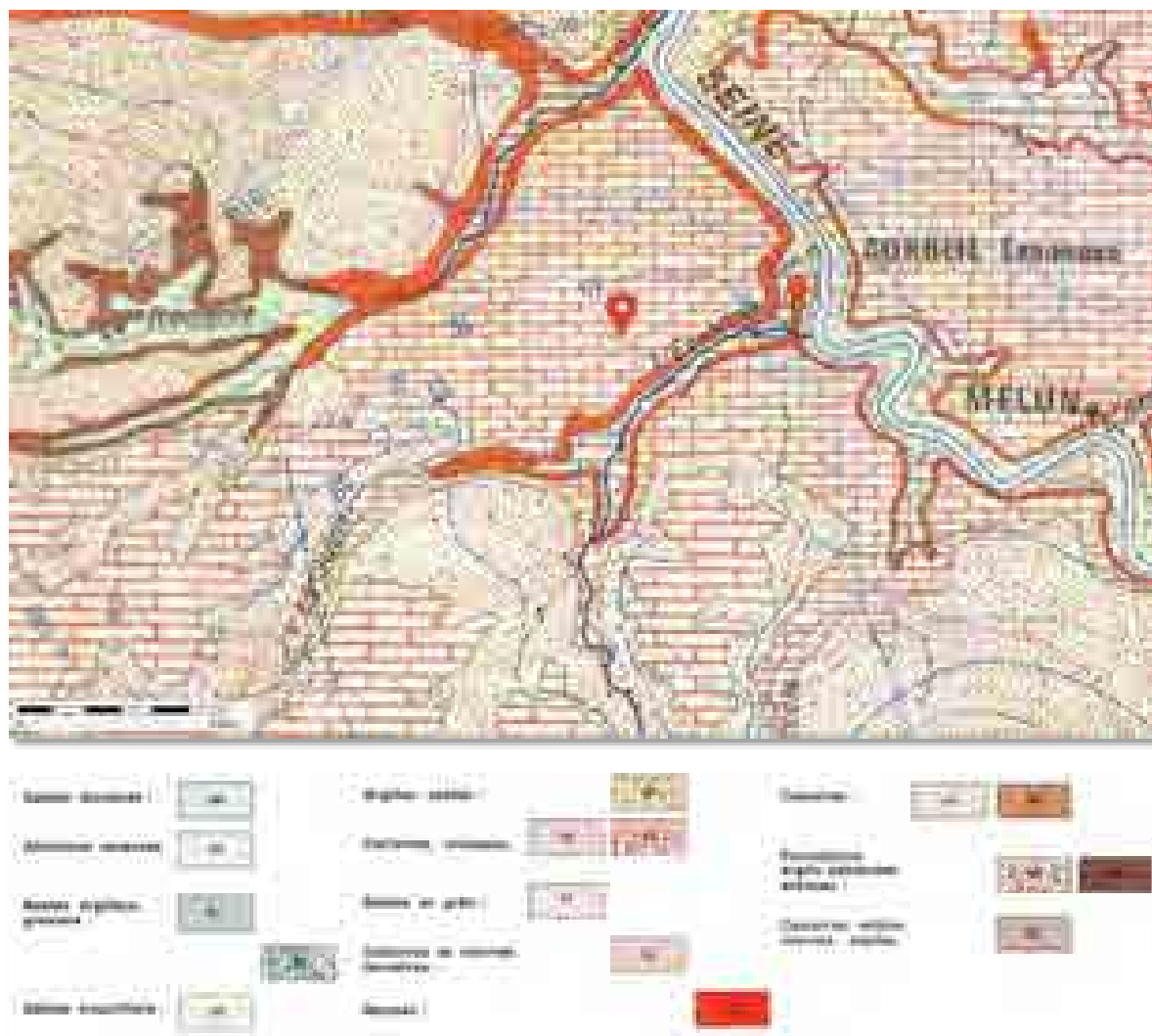
Figure 49: Carte hydrogéologique au 1/200 000 ème , BRGM, SIGES Seine-Normandie.
