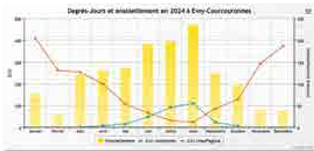
Figure 31. Ensoleillement en 2024, station météo Evry-Courcouronnes, Infoclimat.
