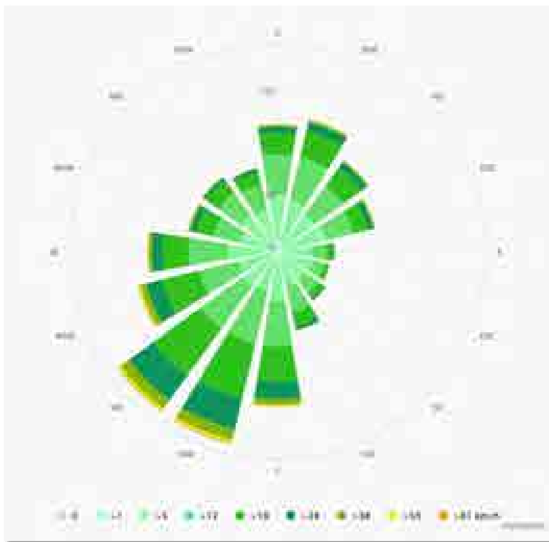
Figure 36 Rose des vents Orly-Athis-Mons, Météoblue.
