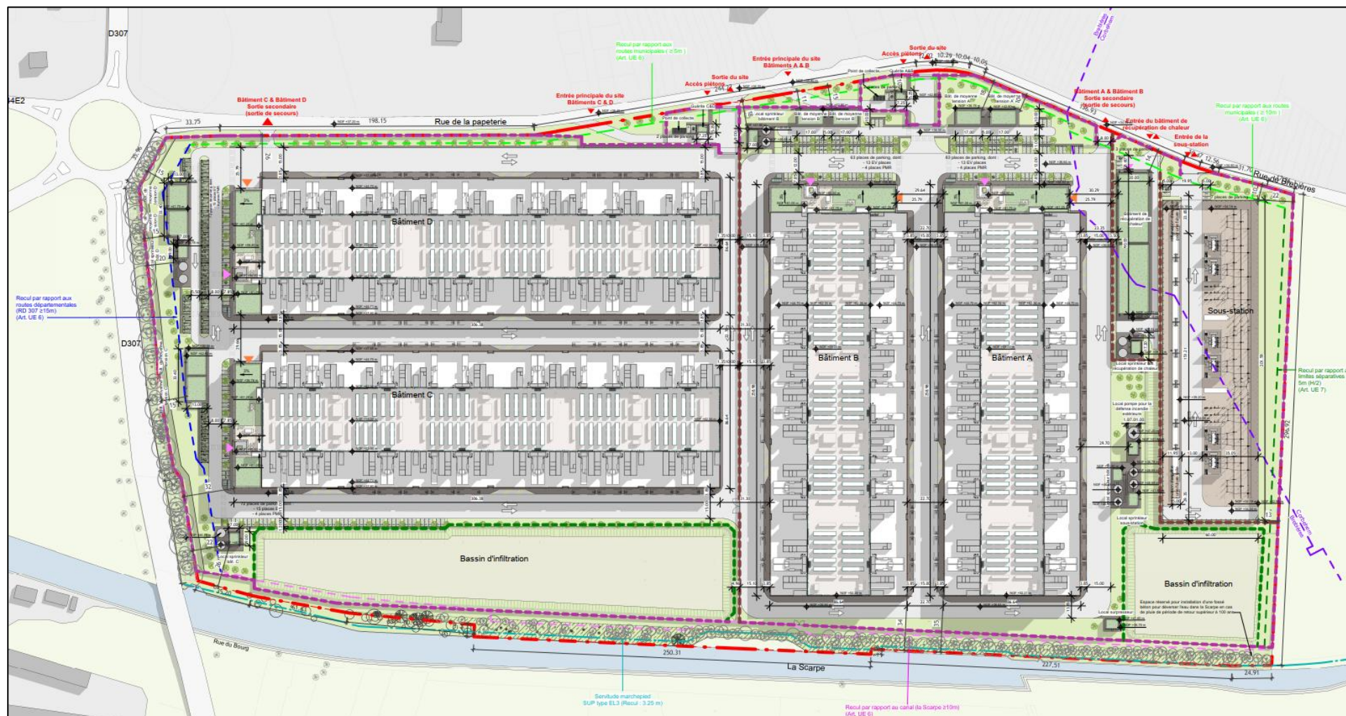
Illustration 5 : Plan de masse du projet LLE01
