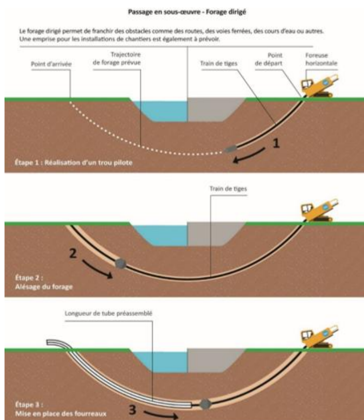
Illustration 12 : Forage dirigé
