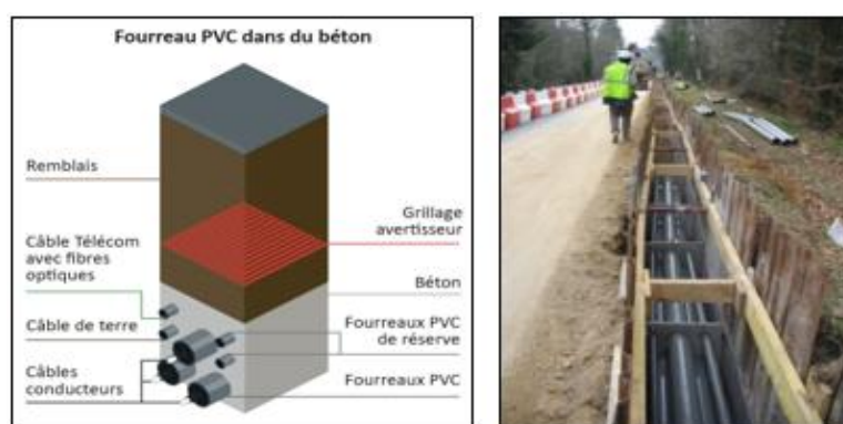
Illustration 9 : Coupe type d'une liaison souterraine en technique PVC 225 000 volts (pose en trèfle)
