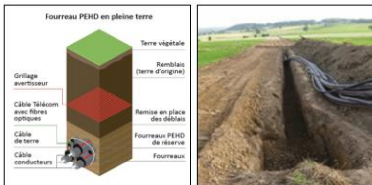
Illustration 8 : Coupe type d'une liaison souterraine en technique PEHD 225 000 volts (pose en trèfle)
