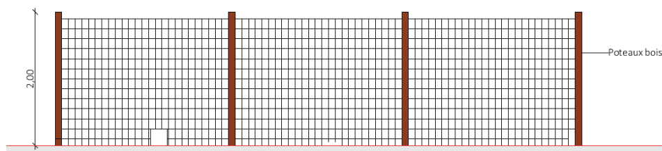
Illustration d'une clôture URSUS avec des passes faunes et des poteaux en bois
