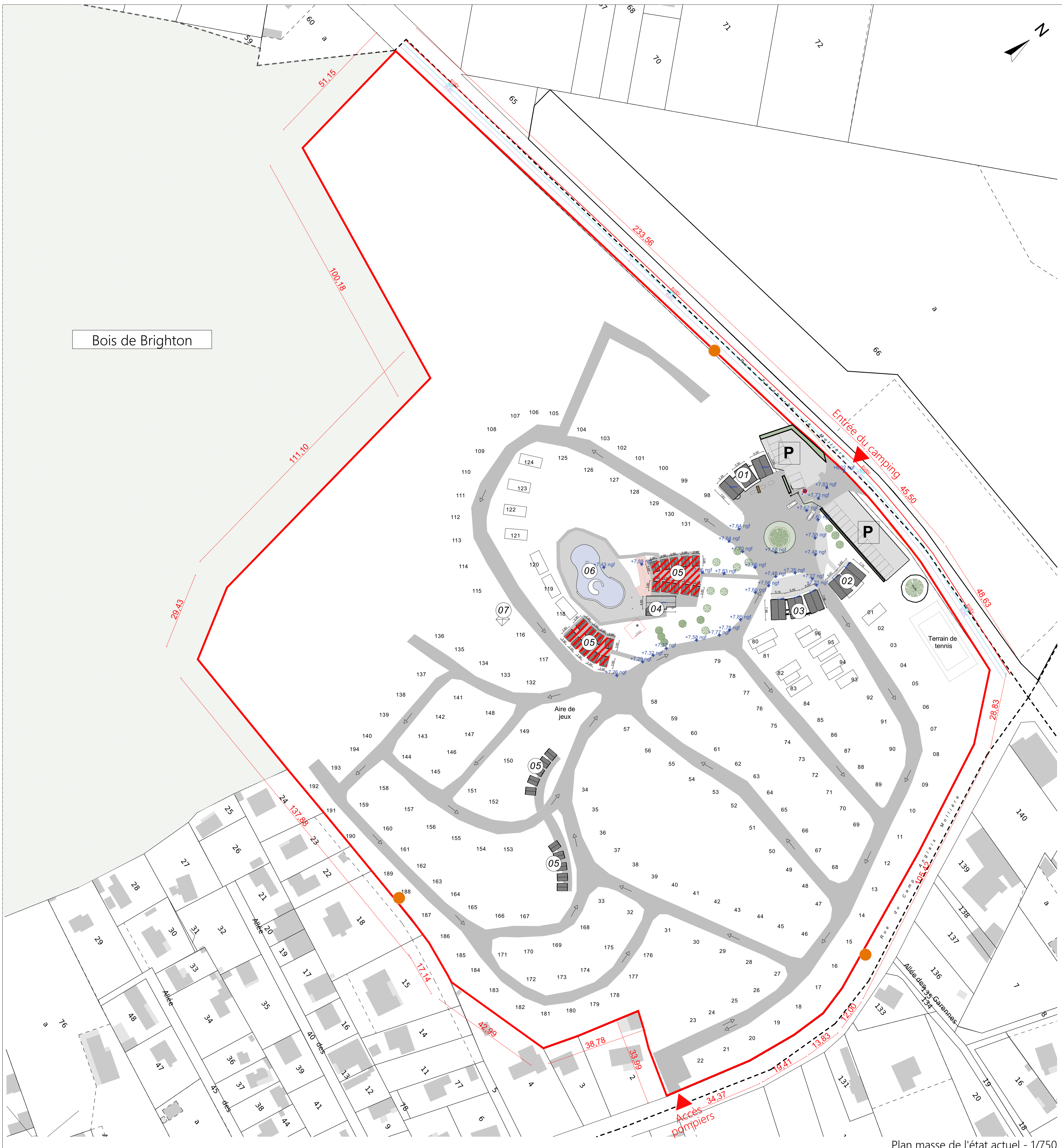
Plan masse de l'état actuel - 1/750
