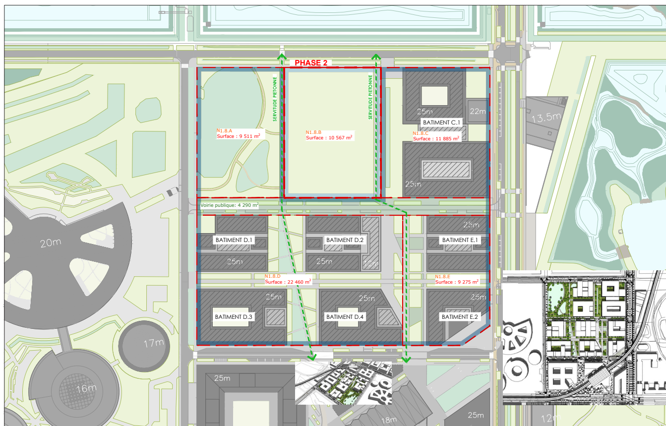
Fig.45 : Plan masse (Agence FRANC, 2026)
