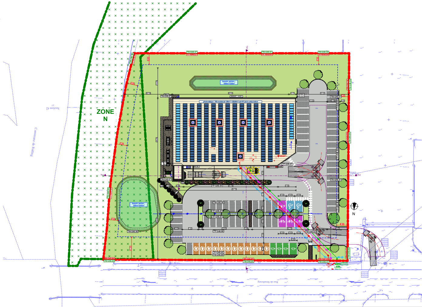
PLAN MASSE PROJET ECH : 1.1000
