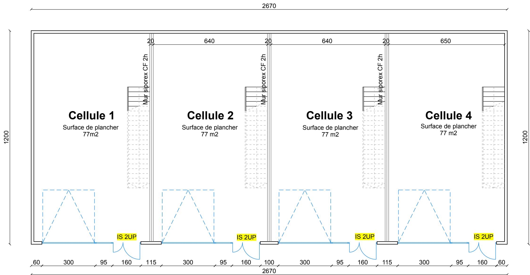
Bâtiment n°3 - Plan rez-de-chaussée
