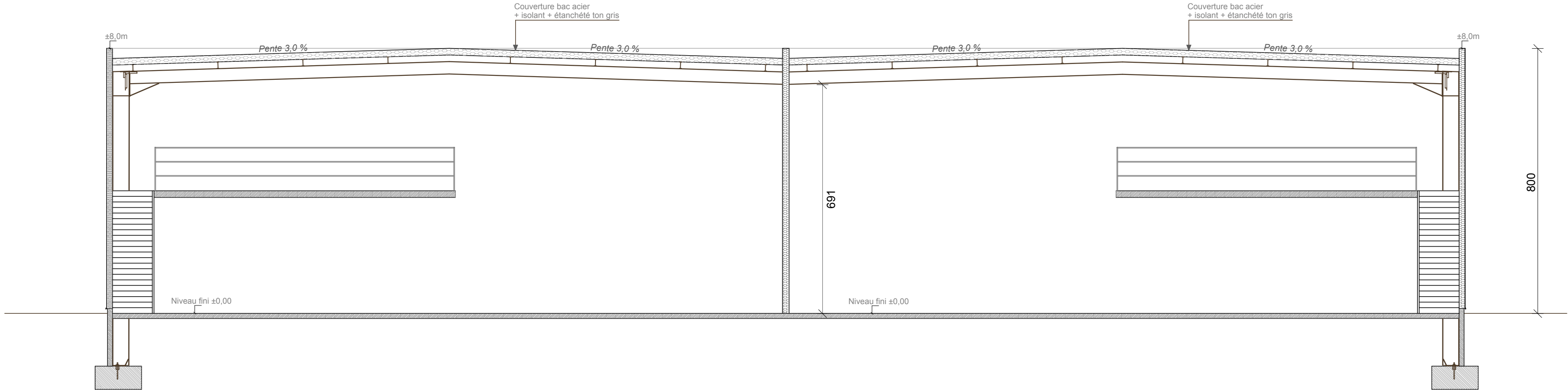
COUPE BB' – Bâtiment n°1
