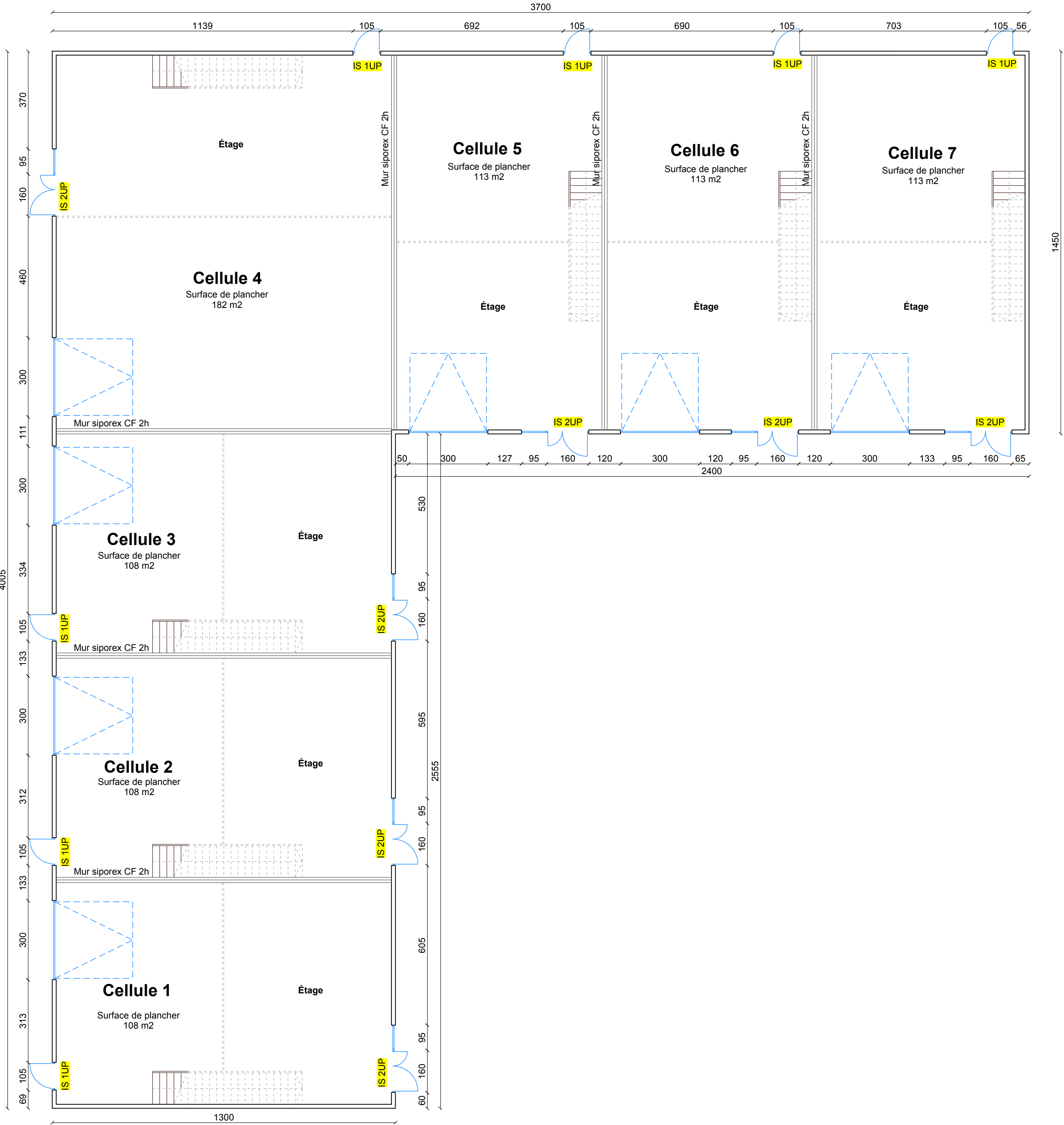
Bâtiment n°2 - Plan rez-de-chaussée
