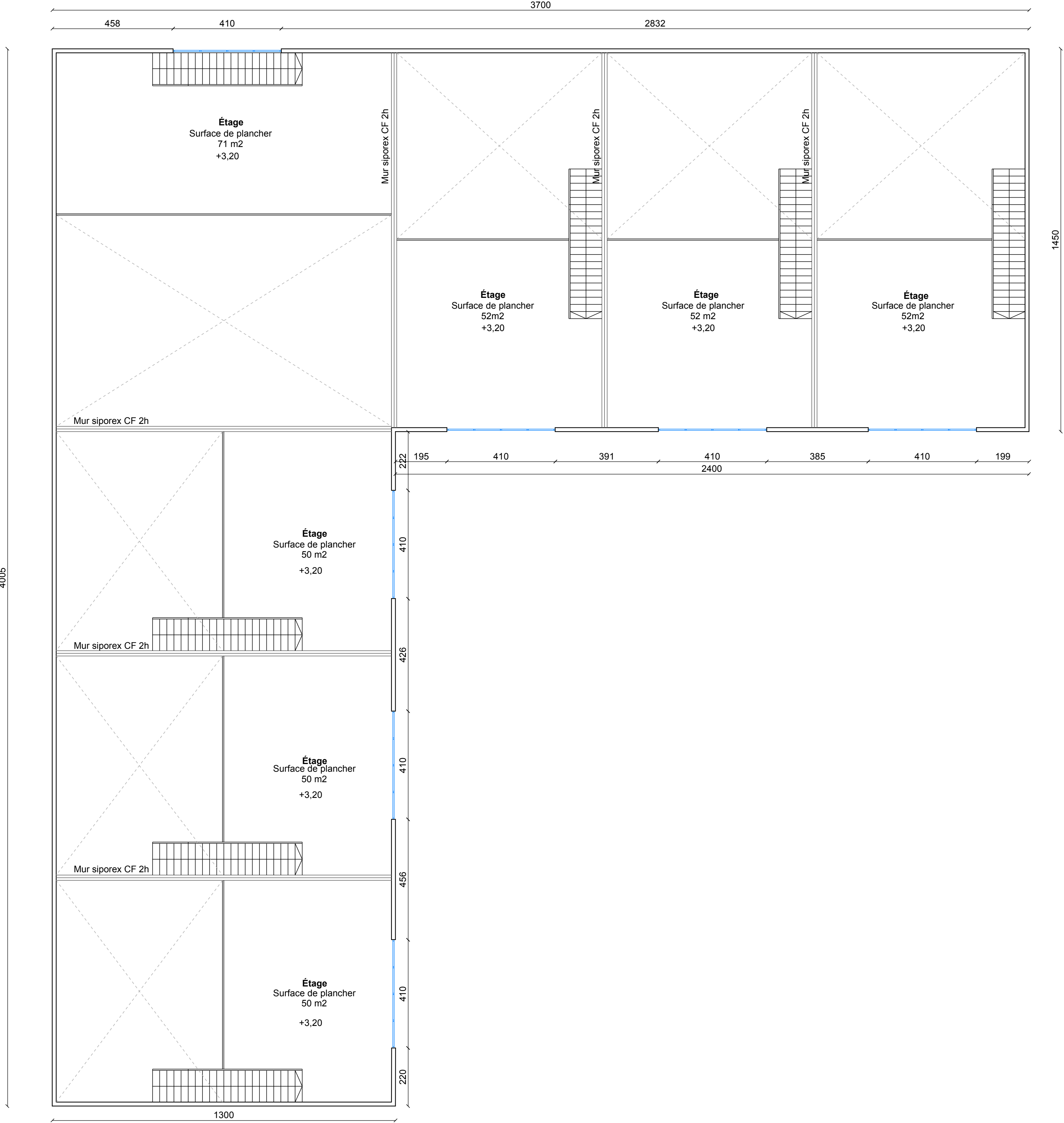
Bâtiment n°2 - Plan étage
