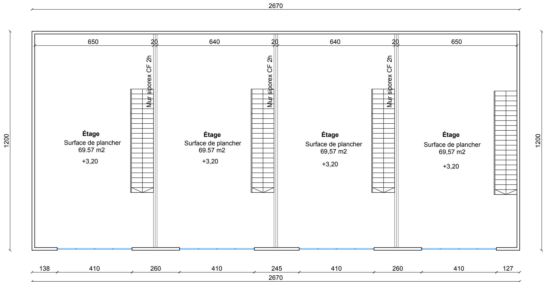
Bâtiment n°3 - Plan étage
