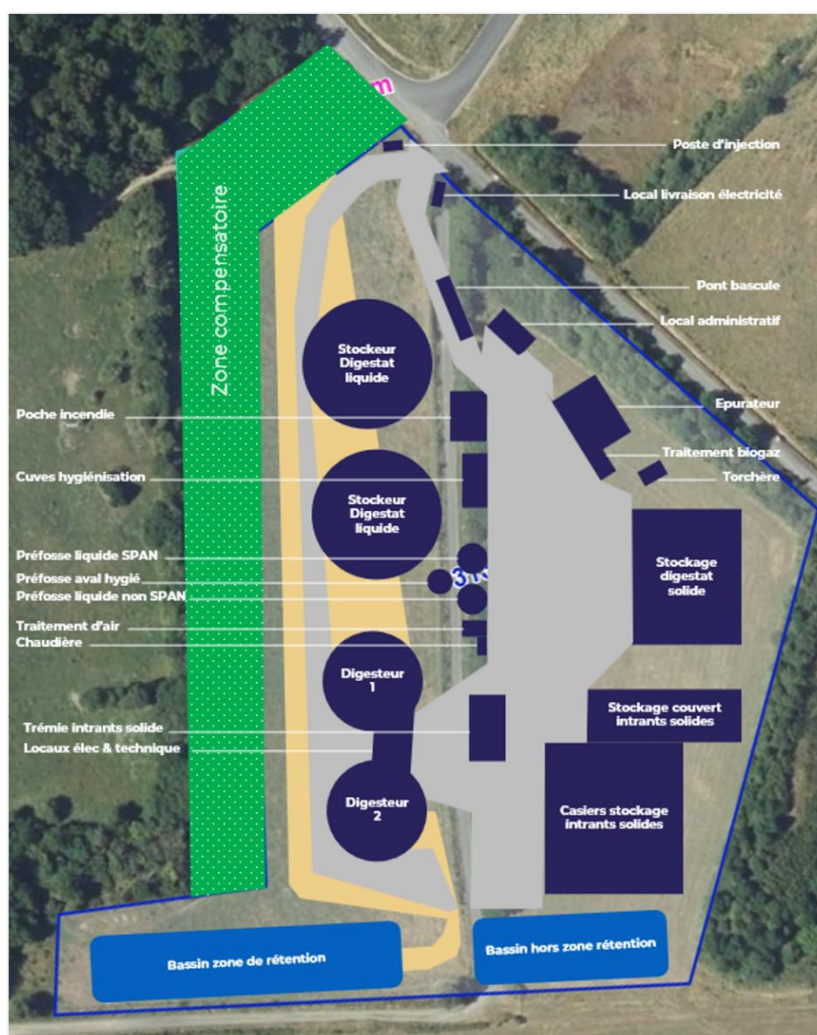
Plan de composition du projet
